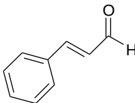
Рис. 1. Коричний альдегід
