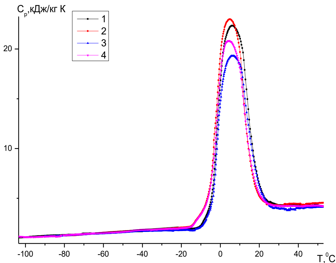
Рис. 1 – Термограми 10% клейстерів:
