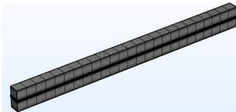
Рис. 2. Розрахункова сітка
