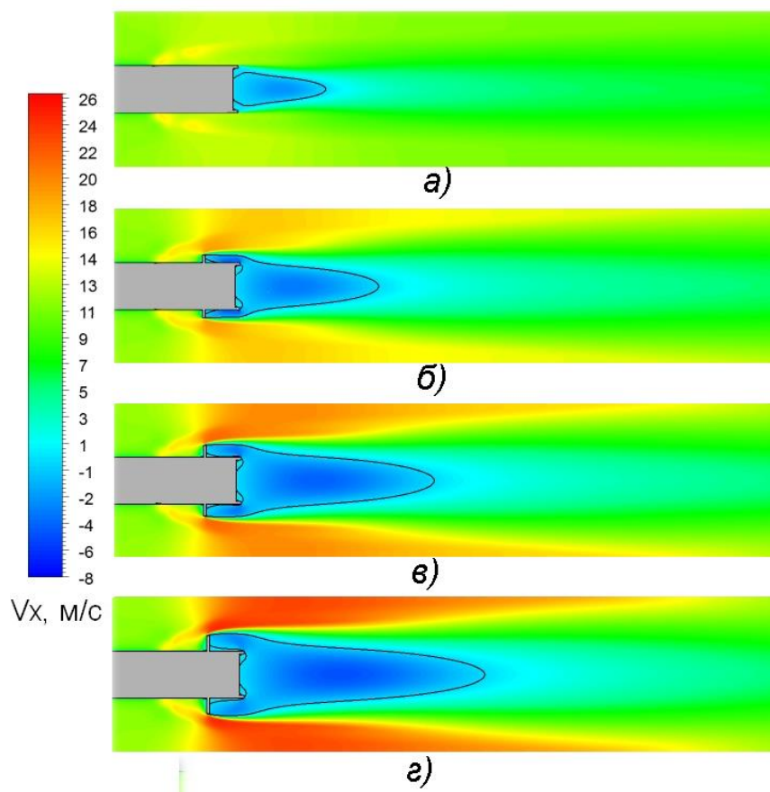
Рис. 3. Поля швидкості V_x в поздовжньому перерізі каналу, що проходить по середині між газоподавальними отворами, без турбулізуючої пластини (а), та з турбулізуючою пластиною різної висоти h_T : (б) – h_T = 5 \cdot 10^{-3}
