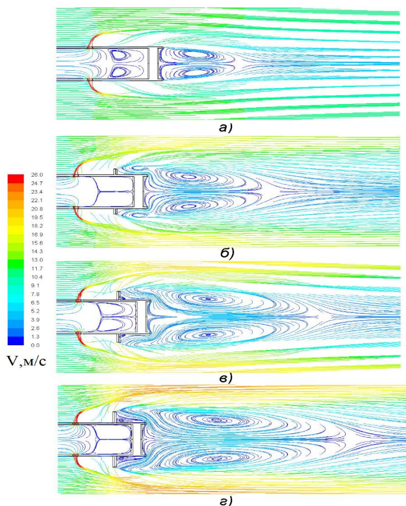
Рис. 2. Картина ліній току в поздовжньому перерізі каналу, що проходить через вісь газоподавальних отворів, без турбулізуючої пластини (а), та з турбулізуючою пластиною різної висоти h_{\text{T}} : (б) – h_{\text{T}} = 5 \cdot 10^{-3} \text{ м} , (в) – h_{\text{T}} = 7,5 \cdot 10^{-3} \text{ м} , (г) – h_{\text{T}} = 10 \cdot 10^{-3} \text{ м}
