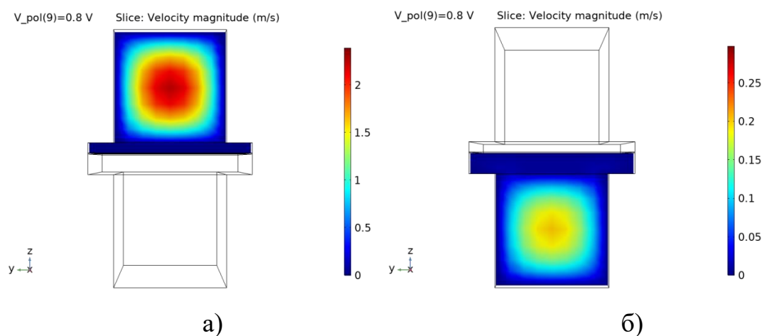
Рис. 3. Розподіл швидкості потоку окислювача (а) та палива (б) у каналах ТОПЕ
