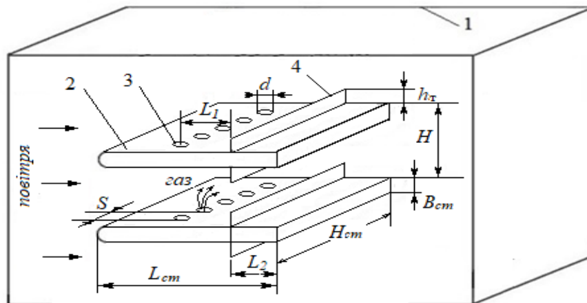
Рис. 1. Схема пальникового пристрою стабілізаторного типу з турбулізуючими пластинами на бічних поверхнях стабілізаторів полум'я: 1 – канал; 2 – стабілізатор полум'я; 3 – газоподавальні отвори; 4 – турбулізуюча пластина.
