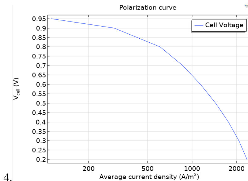
Рис. 4. Поляризаційна крива
