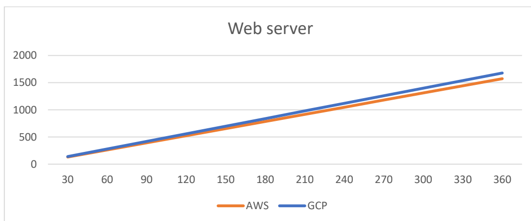
Рис.3 Графік веб-серверів
