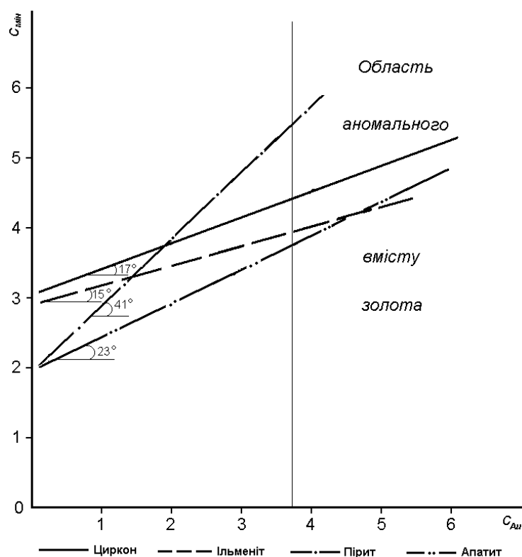
Рис. 2. Графіки зв'язку між вмістами золота та його мінералів-супутників у конгломератах Білокоровицької структури, побудовані за рівняннями лінійної регресії для величини s = \ln(C \cdot 1000) . C – значення вмісту золота (г/т) і мінералів (кг/т) у пробах породи. Кути нахилу графіків до горизонтальної осі визначено як арктангенси їх кутових коефіцієнтів у рівняннях регресії
