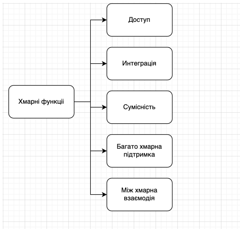
Рис.2. Хмарні функції
