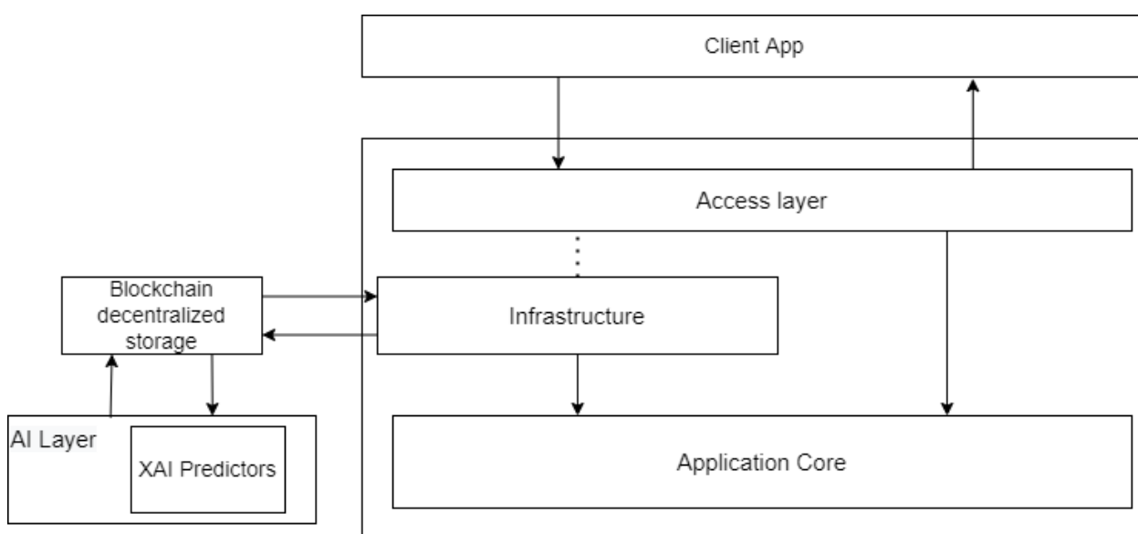
Рис.1. Архітектура рішення
