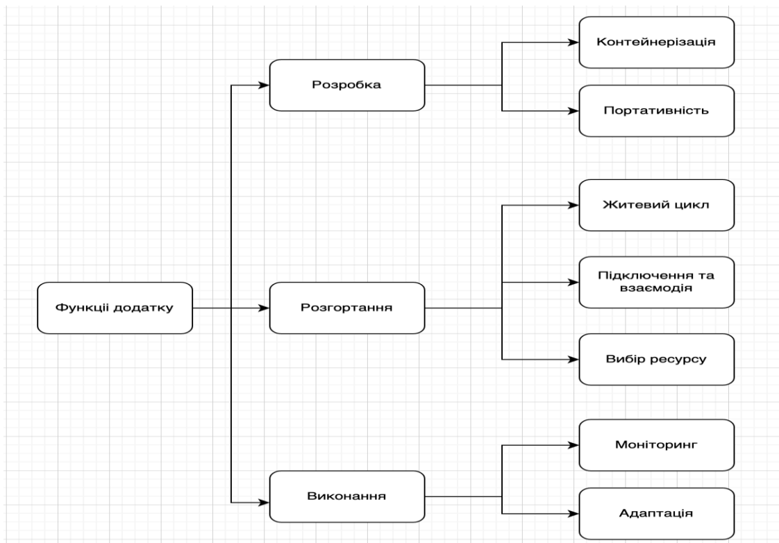
Рис.3. Функції програми
