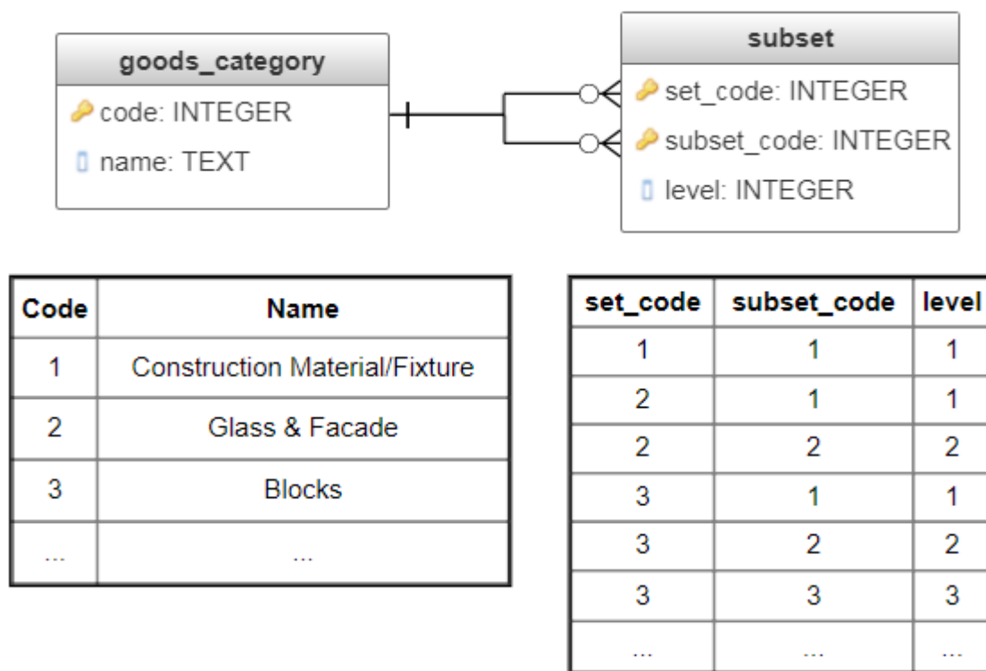
Рис.4. Використання підмножини
