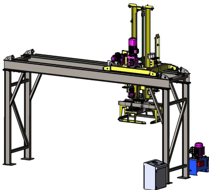
Рис.1 Роботизованих захватів пакетувальника промислового типу
