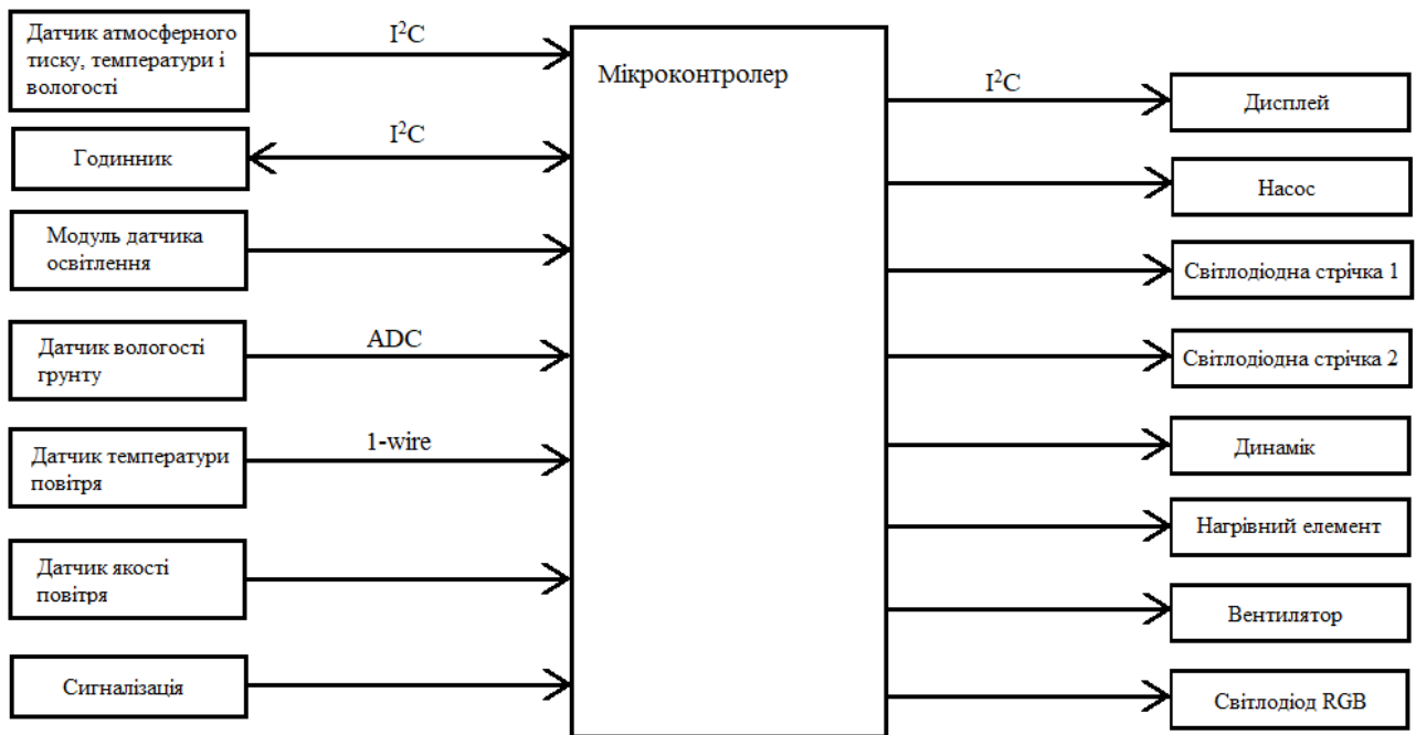
Рис. 1. Структурна схема smart-теплиці
