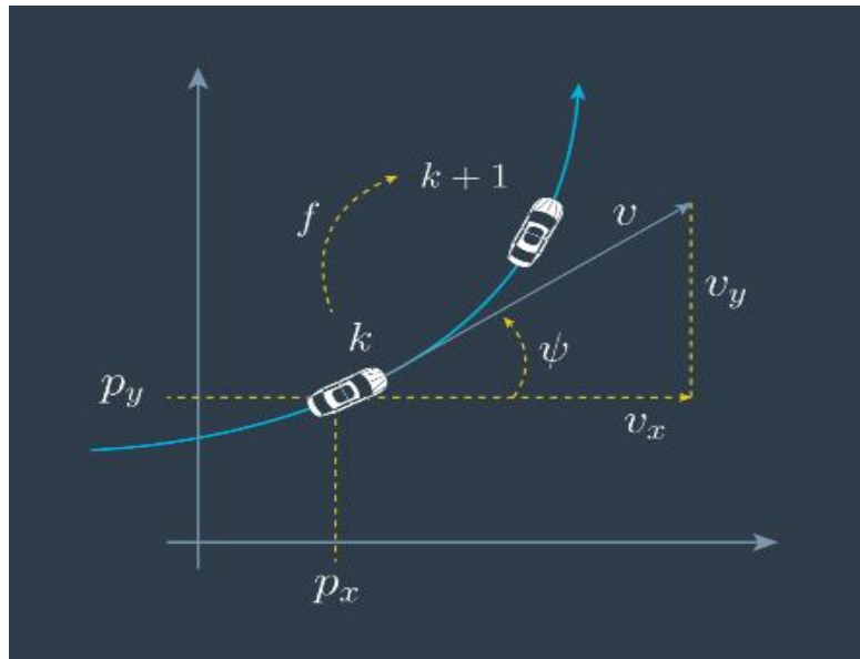
Рис. 1. Характеристики движения транспортного средства согласно модели CTRV [2].
