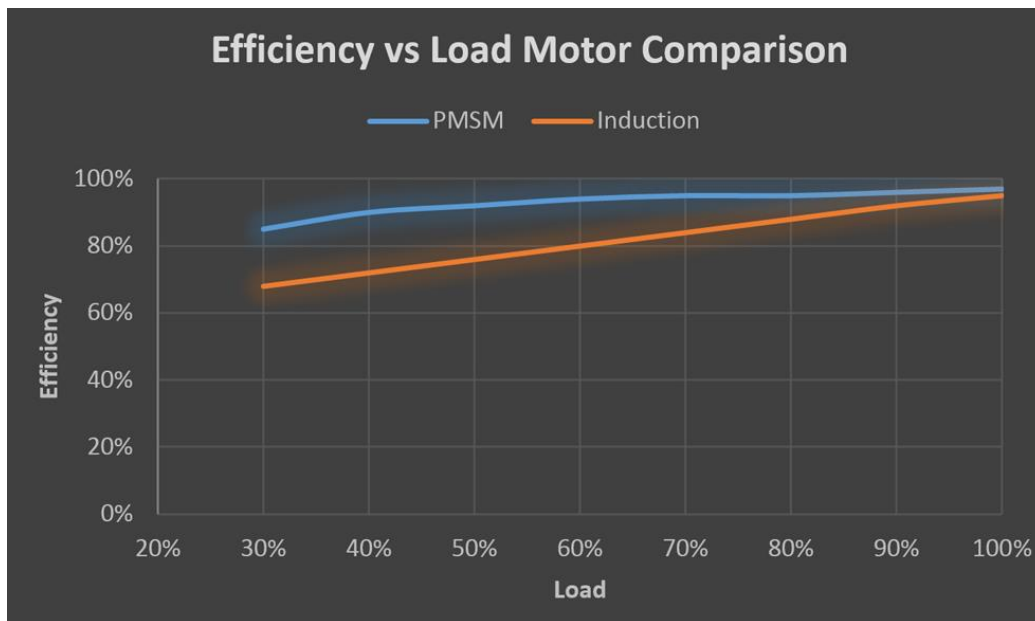
Рис.2 Порівняння ефективності електродвигунів при різному навантаженні [3].
