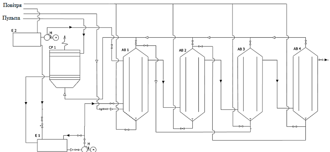
Рис. 1. Схема вилуговування уранових руд
