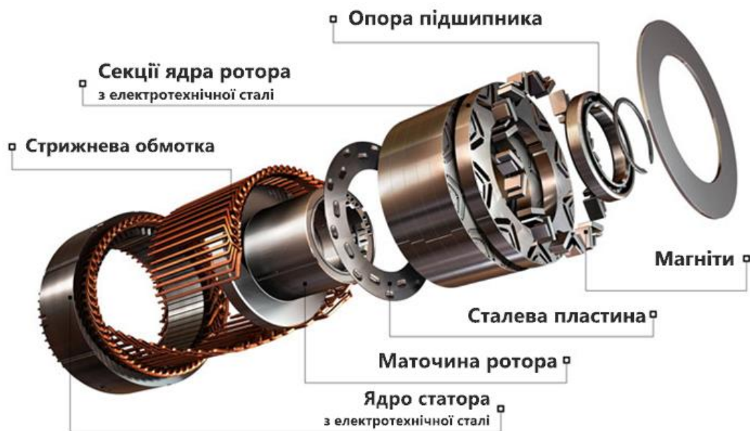
Рис.1 Робочі компоненти синхронного двигуна постійними магнітами [2].
