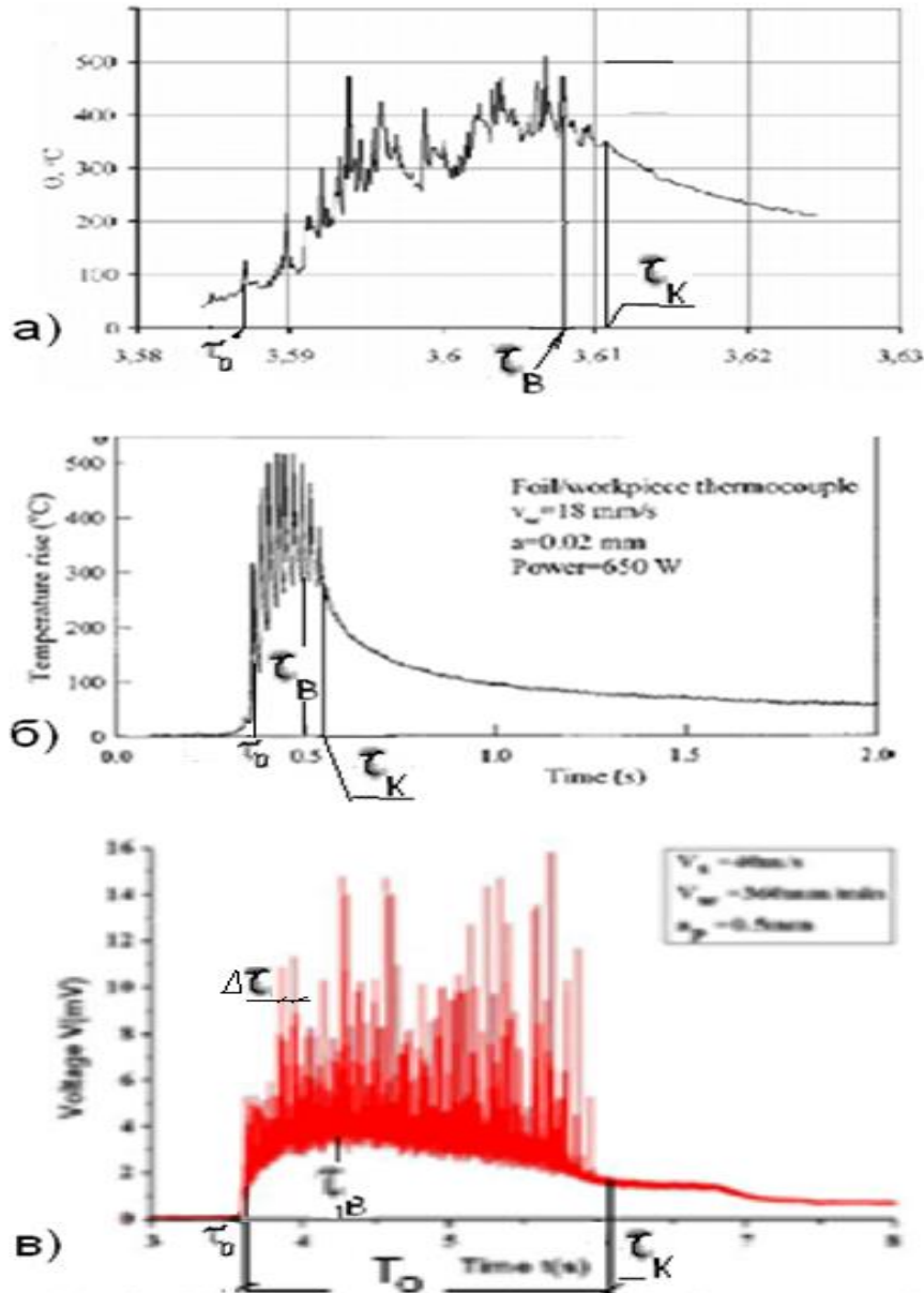
Рис. 1 – Результати вимірювання температури методів шліфування: а) круглого поздовжнього; б) попутного плоского ;в) плоского.
