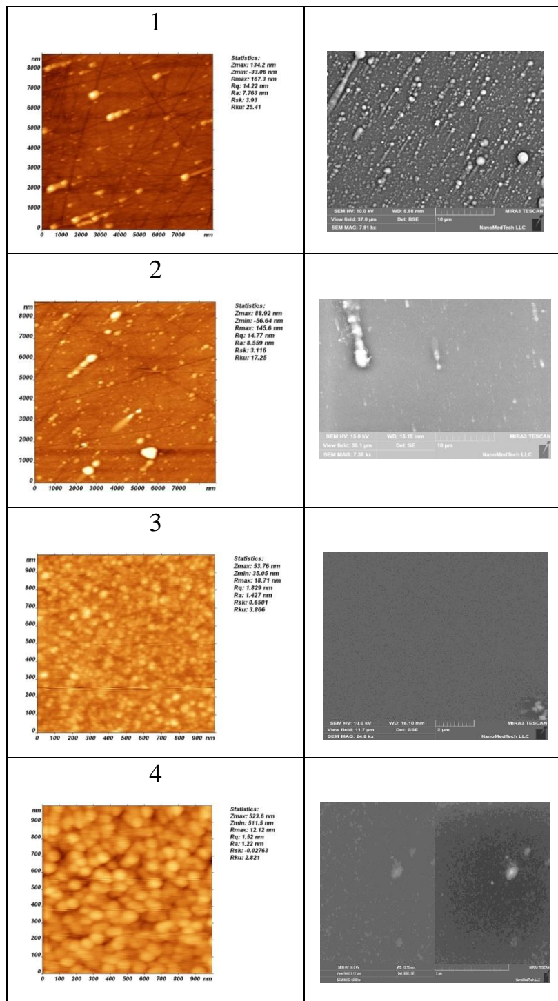
Рис. 2 Рельєф поверхні зразків AlN синтезованих у місці А (2.1, 2.2) і у місці С (2.3, 2.4). 2.1 і 2.3 – поверхня синтезована плазмою ПДП; 2.2 і 2.4 – поверхня синтезована плазмою ПДП з асистуванням її плазмою геліконного джерела (зліва – данні AFM, справа данні SEM)
