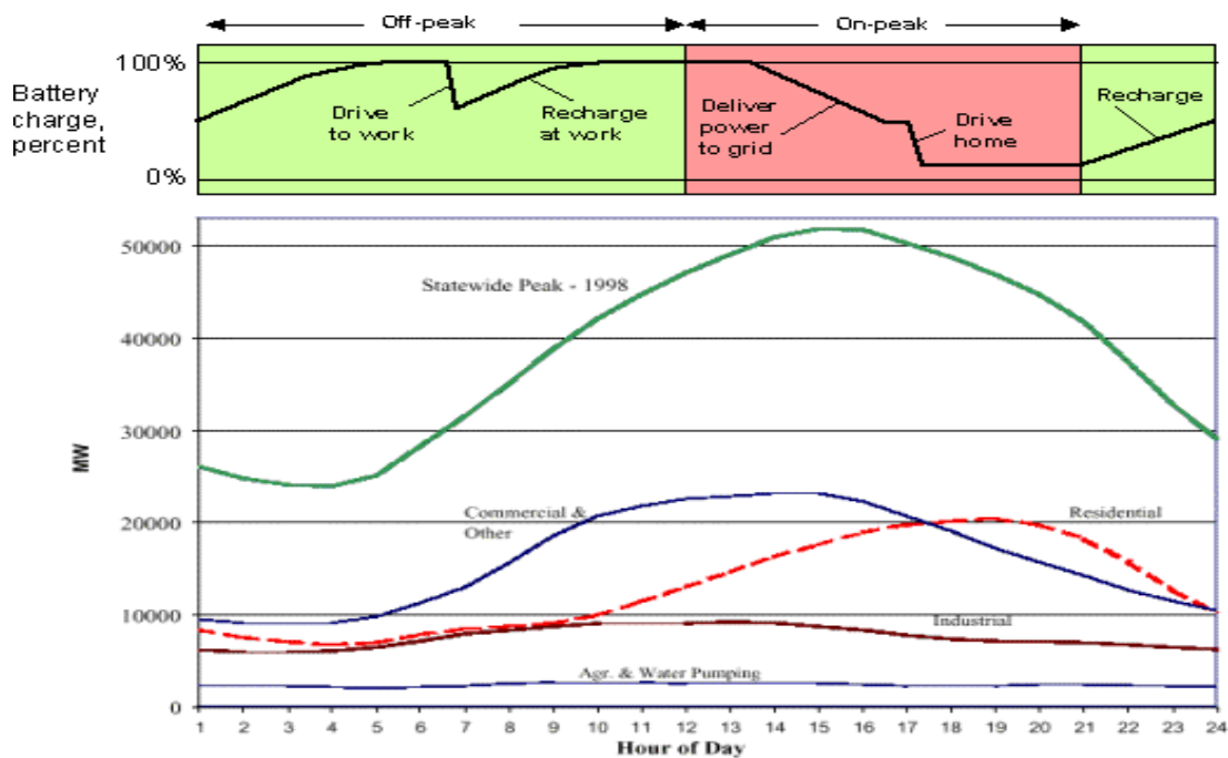
Рис. 2. Суміщення графіку зарядки/віддачі електроенергії електромобілем та добового графіку електричного навантаження енергосистеми.
