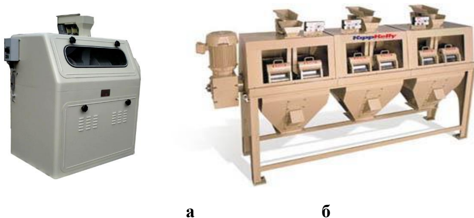
Рис. 2. Крупорізки з двома та шістьма барабанами.
