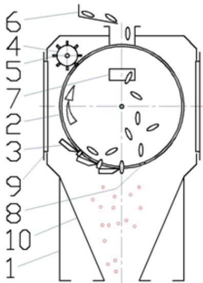
Рис. 1. Схема крупорізки.
