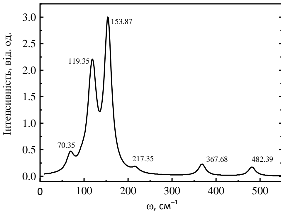
Рис. 3. КР спектр кристала \text{AlSiTe}_3 .
