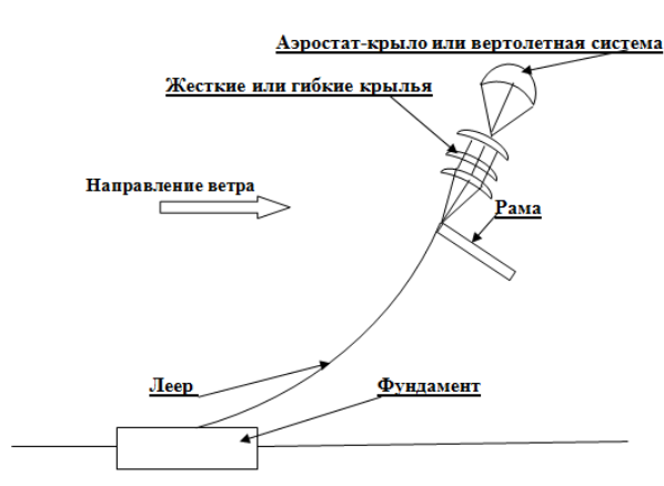
Рисунок 2. Схема безбашенной ветроэлектростанции
