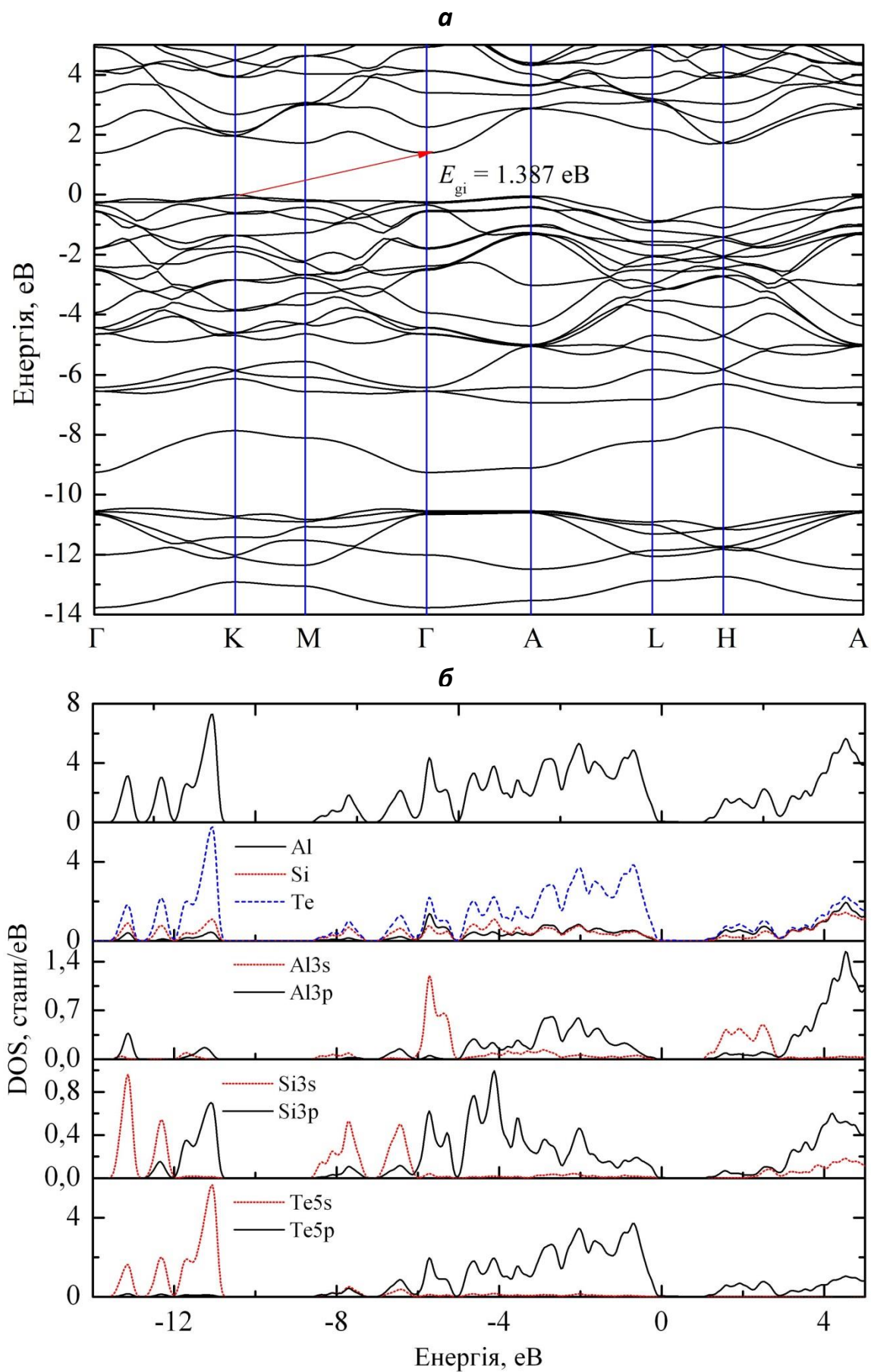
Рис. 2. Електронна структура (а), повна і локальні парціальні густини станів (б) \text{AlSiTe}_3 розраховані гібридним функціоналом HSE06.
