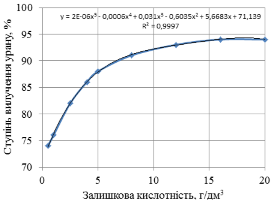
Рис. 4. Залежність ступеня вилучення урану від залишкової кислотності
