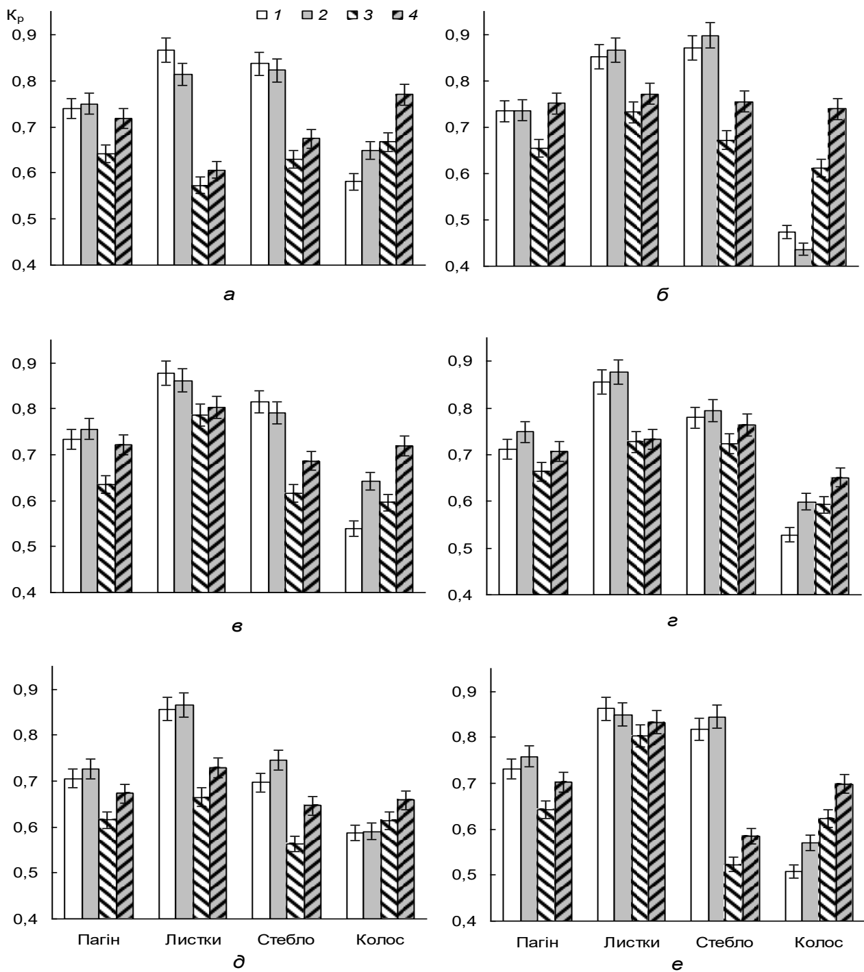
Рис. 1. Коефіцієнти реутилізації азоту з цілого пагона та його частин у процесі наливу зерна у різних сортів пшениці. Тут і на рис. 2: a – Астарта, б – Достаток, в – Наталка, г – Київська остиста, д – Малинівка, е – Куяльник; 1 – високий фон мінерального живлення; 2 – високий фон + позакоренева обробка карбамідом; 3 – низький фон; 4 – низький фон + обробка карбамідом
