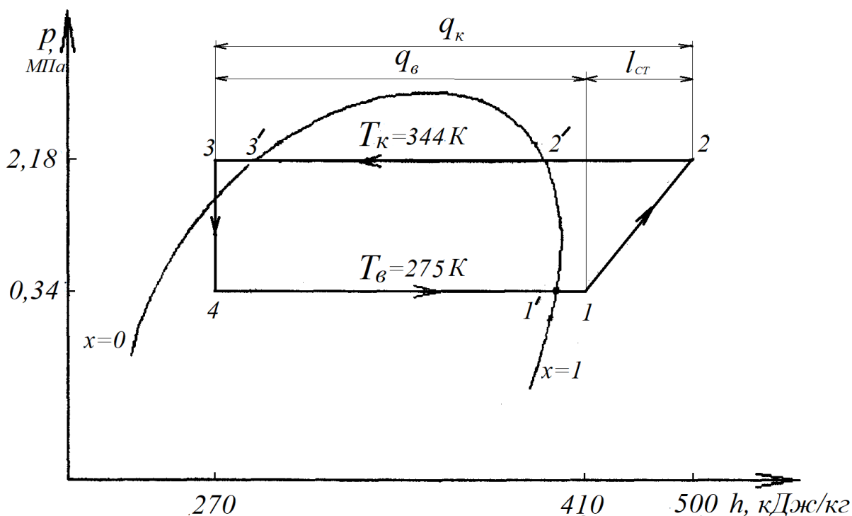
Рис. 1. Цикл ГТН «ґрунт–вода» в p - h -діаграмі
