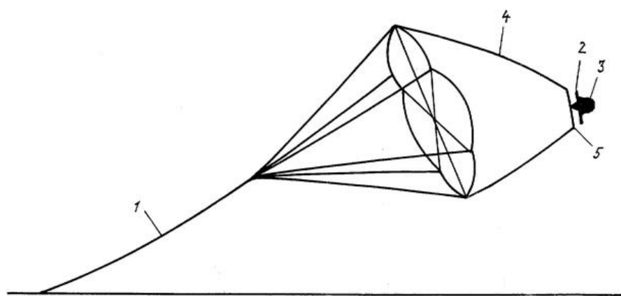
Рисунок 1. Ветроэлектростанция
