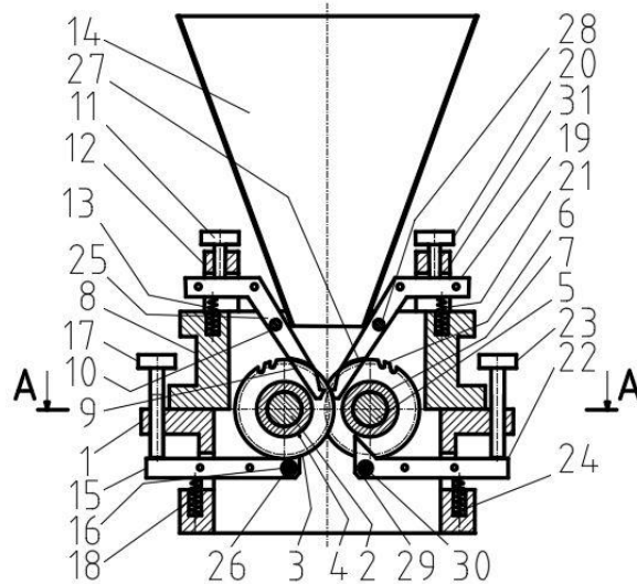
Рис. 4. Схема запропонованої крупорізки.
