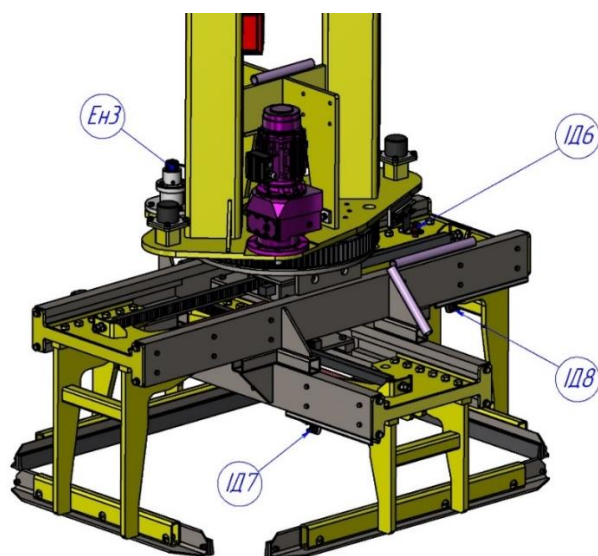
Рис. 2 Схема розміщення датчиків на рухомій колоні та захваті пакетувальника EN3 – Рухома колона ID6 – Кінцевики
