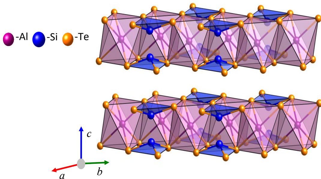
Рис. 1. Кристалічна структура \text{AlSiTe}_3 .
