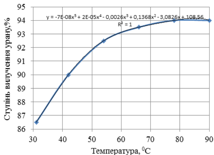
Рис. 3. Залежність ступеня вилучення урану від температури вилуговування
