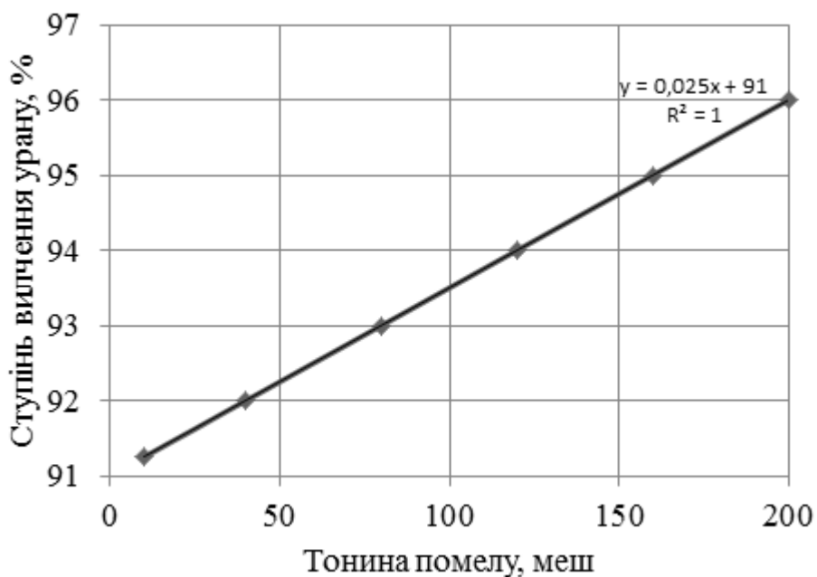
Рис. 5. Залежність ступеня вилучення урану від тонины помелу
