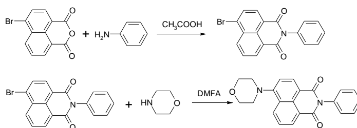
Рисунок 5 – Схема получения 4-морфолино-N-нафталимида по методике 1
