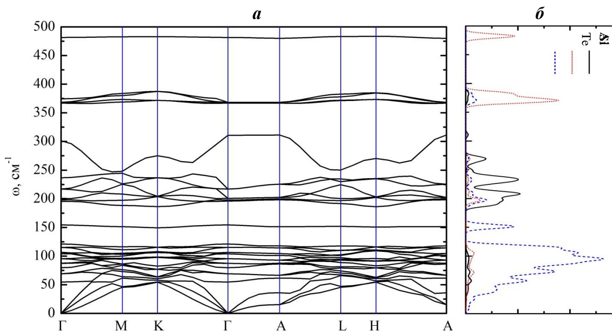
Рис. 4. Дисперсія фононів (а) і проєктовані на атоми густини фононних станів (б) кристала \text{AlSiTe}_3 . зв'язку Al–Te та Si–Te.
