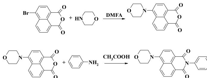
Рисунок 6 – Схема получения 4-морфолино-N-нафталимида по методике 2
