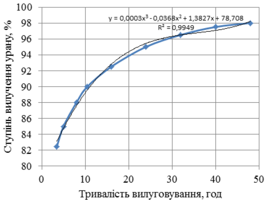
Рис. 2. Залежність ступеня вилучення урану від часу вилуговування
