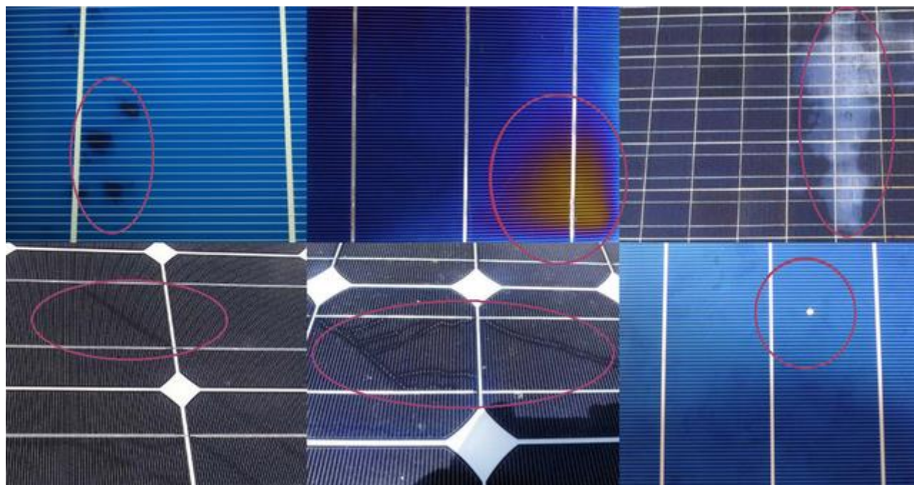
Рис.1. Дефекти сонячних панелей (зліва направо): темні та жовті плями, деламінація; " Сліди равлика", біла пляма від витоку пасти
