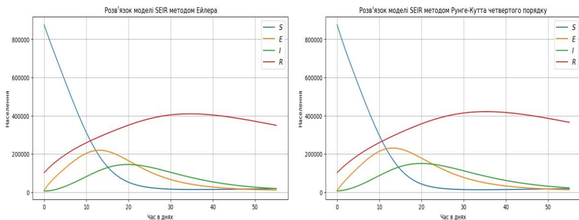
Рис. 1. Результат моделювання методів Ейлера та Рунге–Кутта.
