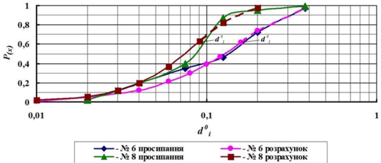
Мал. 1. Інтегральні криві розподілу пор в зразках № 6 і № 8
