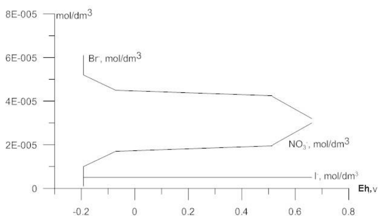
Рис. 1. Графік залежності Eh від вмісту Br - та NO 3 - при незмінному вмісті I - .
