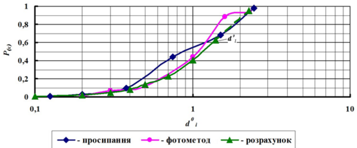
Мал. 2. Інтегральні криві розподілу пор в зразку № 2
