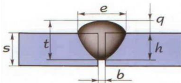
Рис. 1 – Геометричні параметри стикового зварного шва
