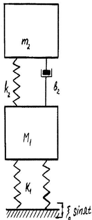
Рис. 1 – Розрахункова схема
