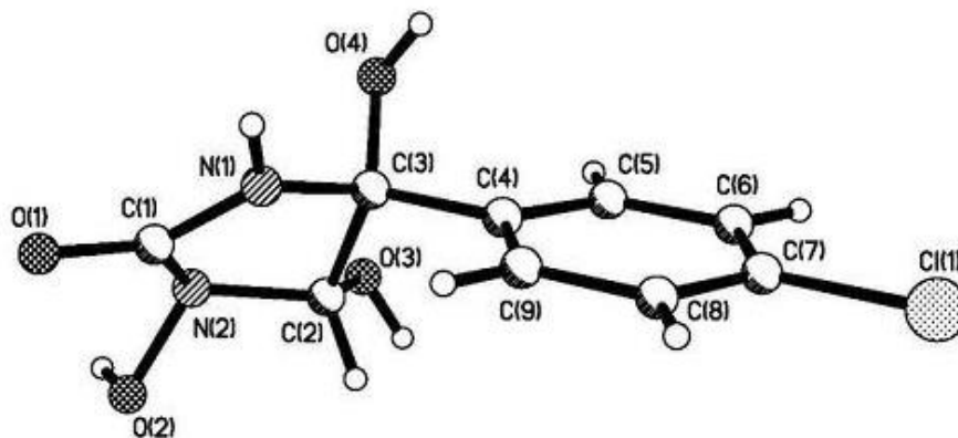
Рис. 1. Будова 3,4,5-тригідрокси-5-(4-хлорофеніл)імідазолідин-2-ону 2d за даними РСА
