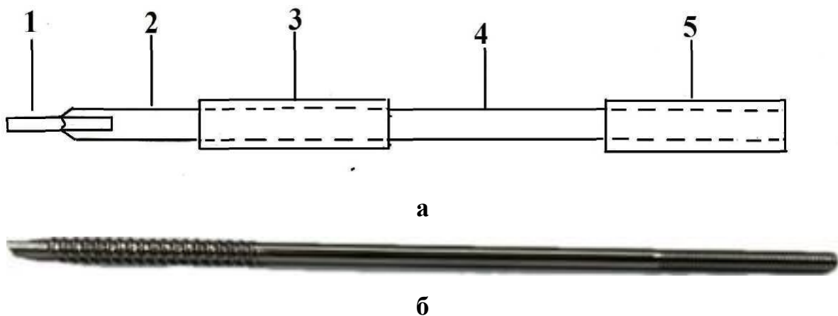
Рис. 1. Схематичне зображення стрижня для компресійного остеосинтеза переломів тіла ключиці (а) : 1- отвір для направляючої спиці, 2- свердло, 3-направляюча різьба, 4- тіло, 5- різьба для компресійної гайки; (б): натуральне зображення стрижня.
