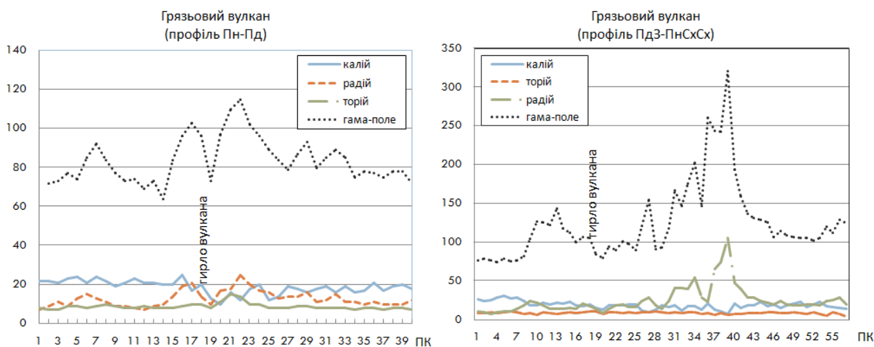
Рис. 3. Розподіл радіоактивних елементів та інтенсивність гама-поля в зоні грязьового вулкану (калій, %; радій, 10^{-3} %; торій, 10^{-3} %; гама-поле, імп/ 10^1 с)
