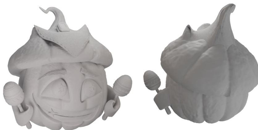
Рис. 5 Текстурування «Джека»
