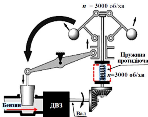
Рис. 2. Схема моделі регулятора Уайта
