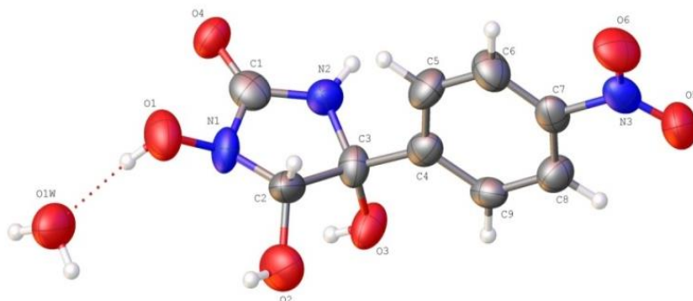
Рис. 2. Молекулярна структура моногідрату 3,4,5-тригідрокси-5-(4-нітрофеніл)імідазолідин-2-ону 2g відповідно РСА
