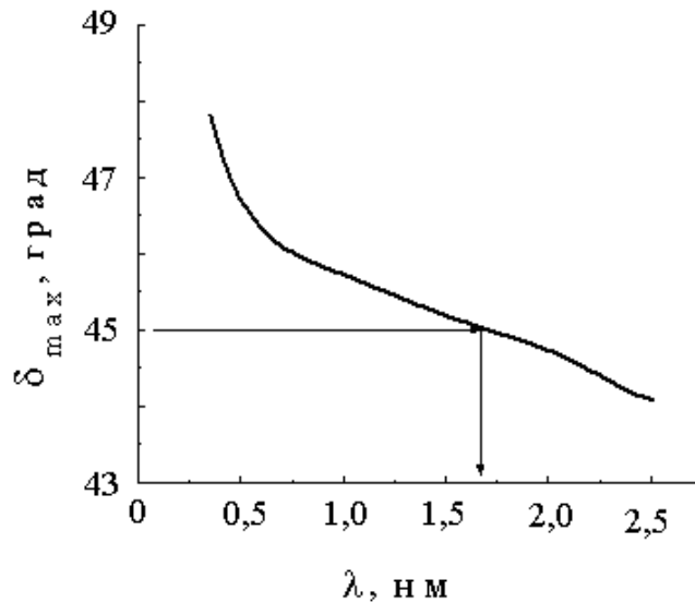
Рис. 3. Залежність \delta_{\max} від довжини хвилі для скла К8. Стрілкою показана довгохвильова границя роботи чверть хвильових ромбів Френеля,
