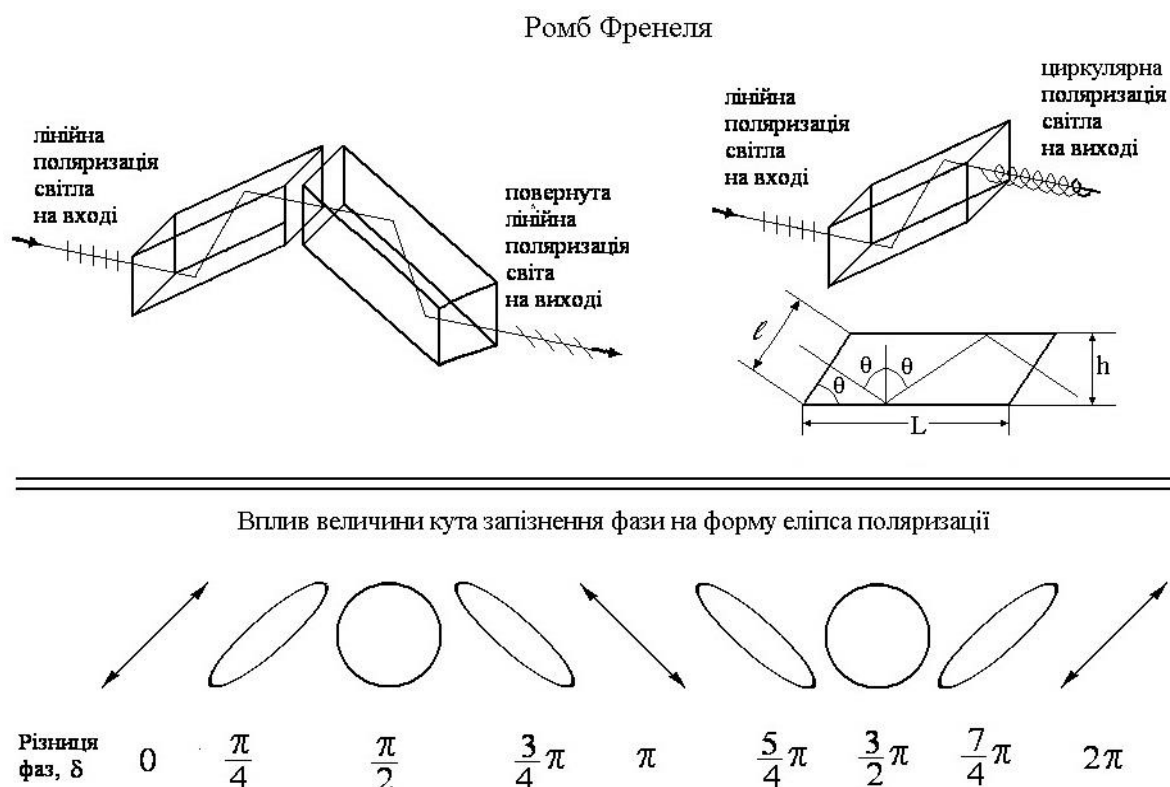
Рис. 1. Ілюстрація впливу ромбів Френеля на стан поляризації світла
