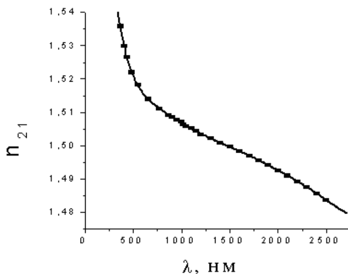
Рис. 2. Дисперсія показника заломлення скла К8 [7] (точки). Суцільна лінія апроксимація поліномом шостого степеня.
