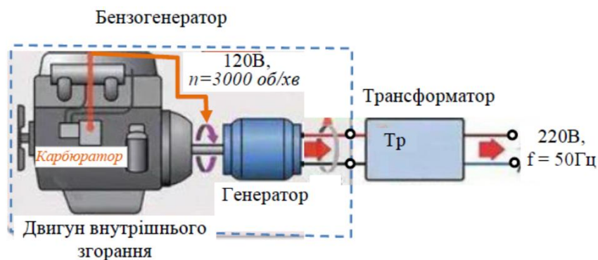
Рис. 1. Узагальнена блок-схема бензинового генератора
