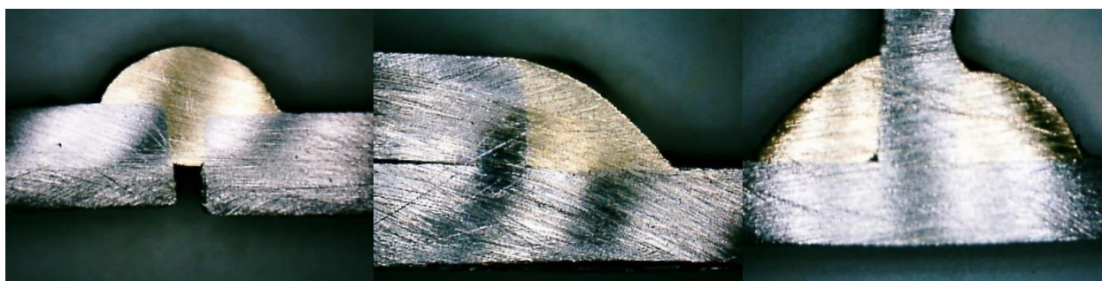
Рис. 4 – Поперечні перерізи зварних швів
