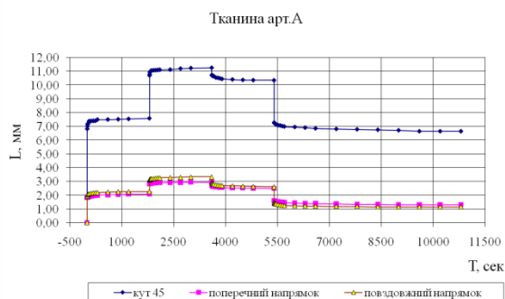
Рис. 4. Статичний модуль пружності. Зразок полотна А (бавовна 100%)
