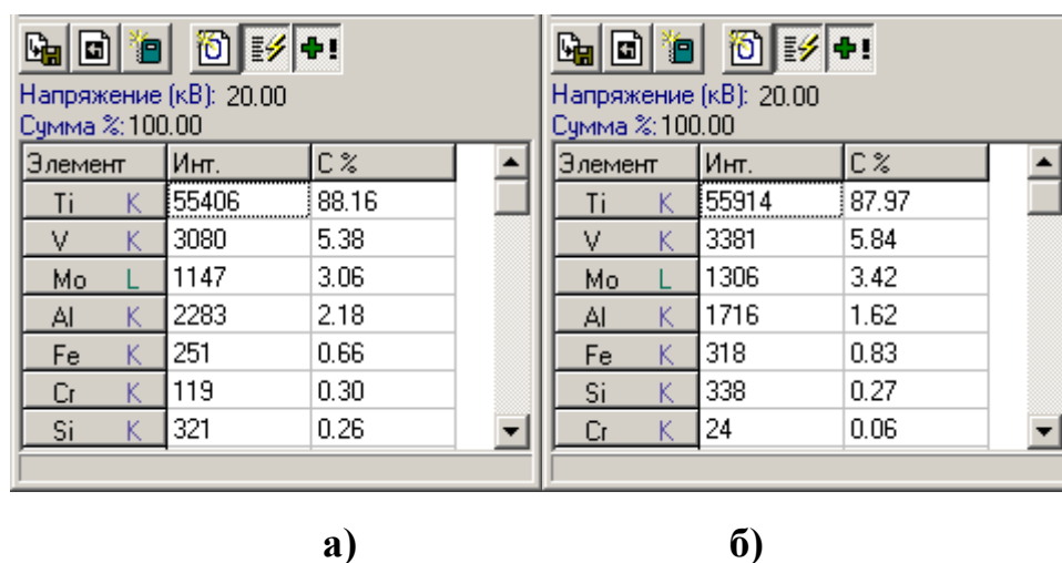
Рис. 2. Хімічний склад \alpha -фази (а) та \beta -фази (б) при старінні 400°C
