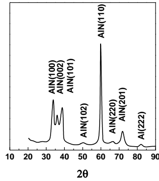
Рис. 2. Дифрактограма системи AlN/Д16.
