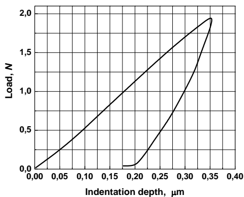
Рис. 4. Криві навантаження/розвантаження наноіндентації.
