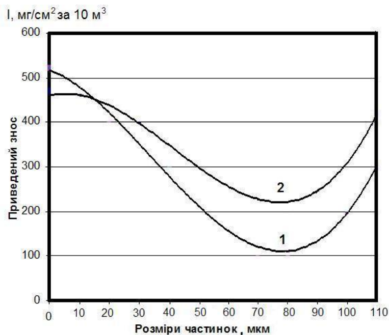
Рис. 1. Залежність зносостійкості КЕП системи Ni-TiC після дифузійного хромування при навантаженні 10Н (1) і 20Н (2).
