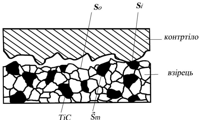
Рис. 2. Схема розташування частинок TiC у поверхневому шарі КЕП
