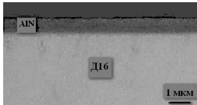
Рис. 1. Спостереження поперечного перерізу покриття AlN/Д16.
