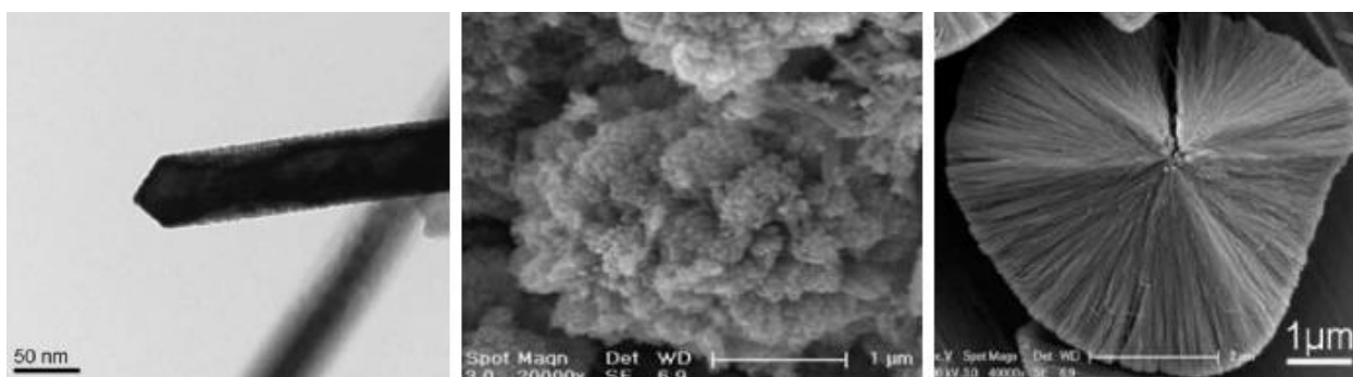
Рисунок. 2. Зображення наночастинок рутилу \text{TiO}_2 в форматі 3D: наностержні та наноквітки; сферична частинка сформована з наностержнів рутилу зорієнтованих радіально від центру до поверхні.
