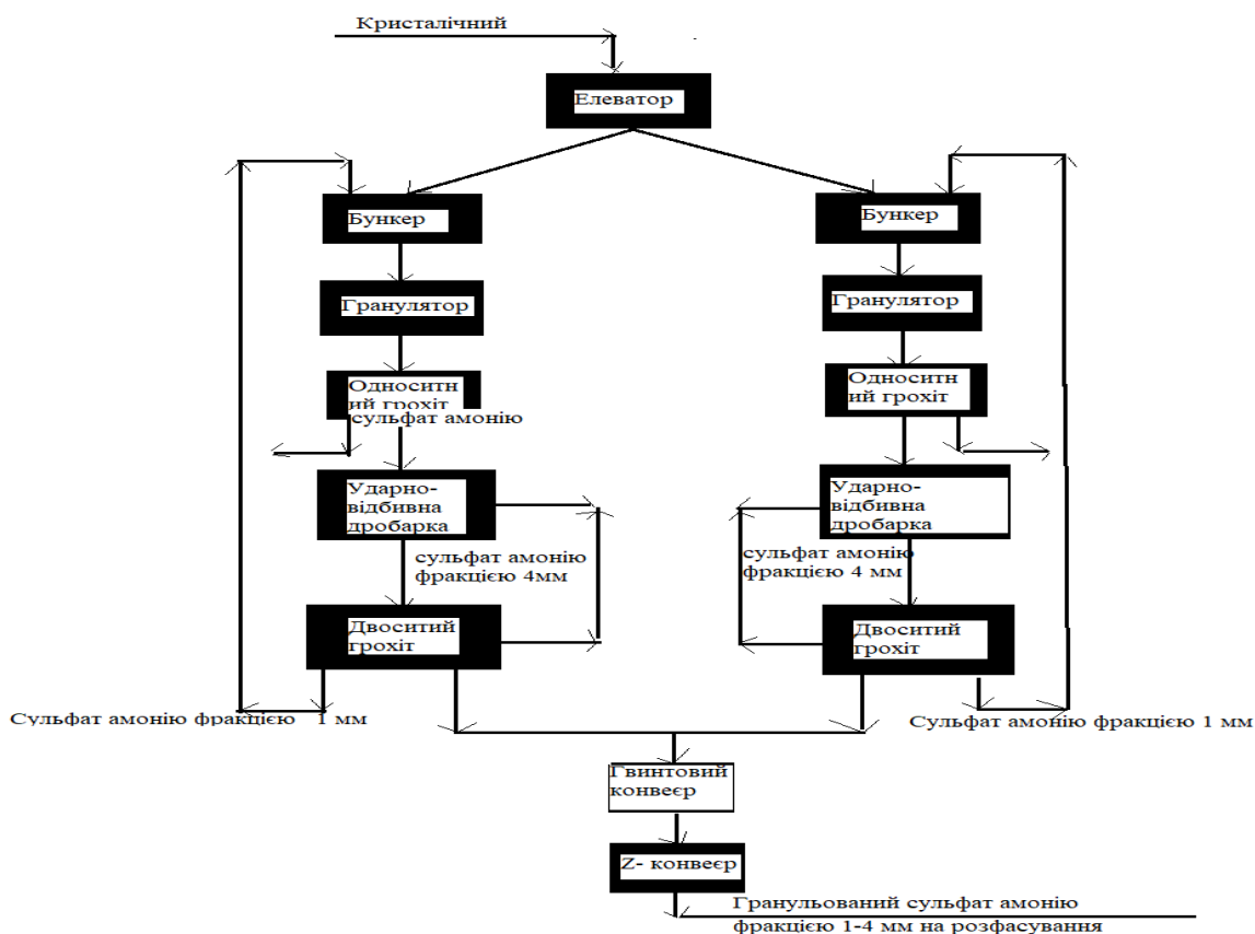
Рис. 4. Блок-схема основного обладнання установки грануляції кристалічного сульфату амонію методом компактування
