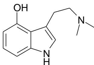
Рис. 6. Псилоцин
