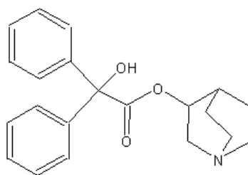
Рис. 5. Хінуклідил-3-бензилат
