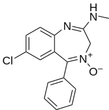
Рис. 14. Хлордіазепоксид
