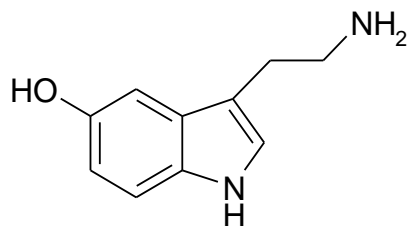
Рис. 3. Серотонін
