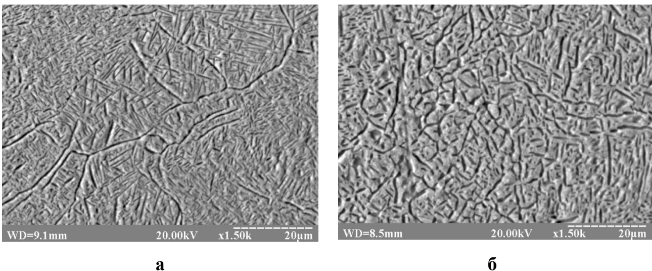
Рис. 3. Мікроструктура титанового сплаву VT22 після гартування t = 750^{\circ}\text{C} та старіння t = 500^{\circ}\text{C} (а), t = 600^{\circ}\text{C} (б), \times 1500
