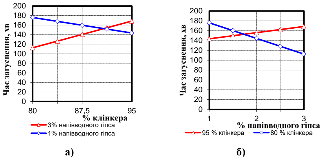
Рис. 3. Залежність часу загуснення до консистенції 30 Вс від вмісту напівводного гіпса та % клінкера в цементі (а), залежність часу загуснення до консистенції 30 Вс від % клінкера в цементі та вмісту напівводного гіпса (б).
