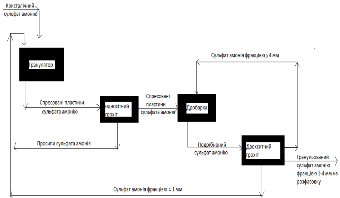
Рис. 2. Блок-схема компактування та подрібнення сульфату амонію
