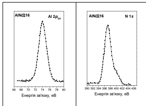
Рис. 3. Енергетичне положення електронних ліній Al 2p і N 1s в РФЕС спектрах.
