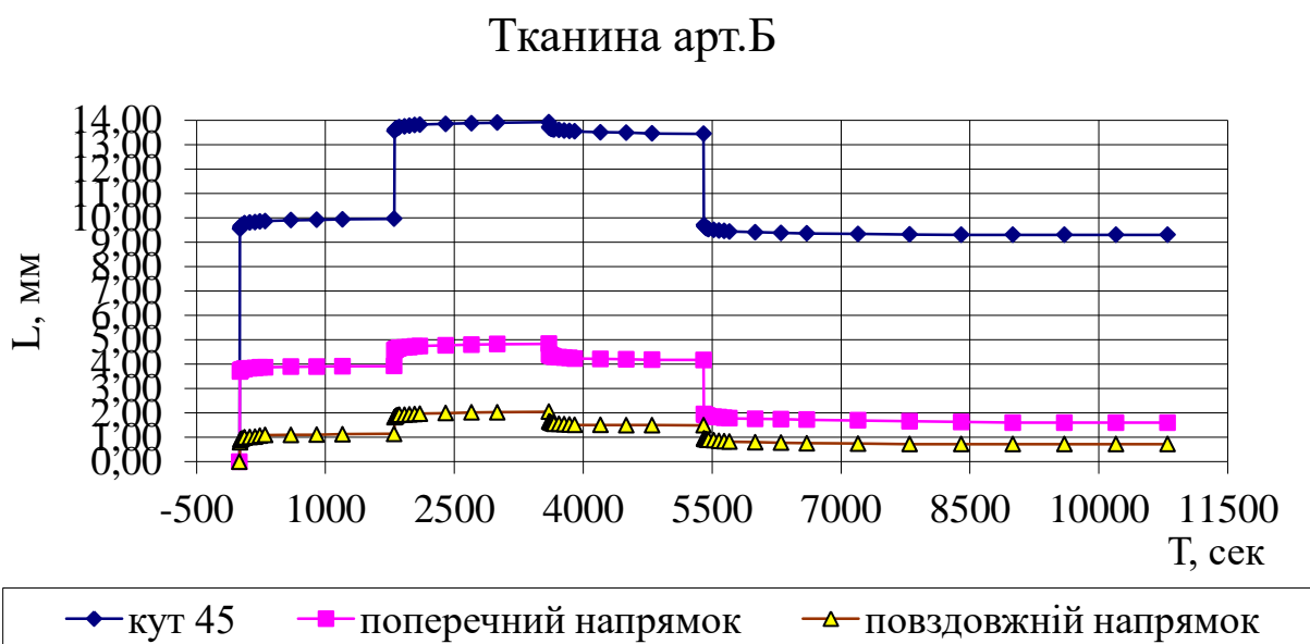
Рис. 5. Статичний модуль пружності. Зразок полотна Б (бавовна 50%, віскоза 50%)
