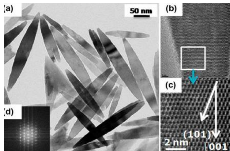
Рисунок. 1. Наночастинки анатазу еліпсоїдної морфології (а); виділена ділянка поверхні окремої наночастинки (b-c); електроннограма матеріалу.
