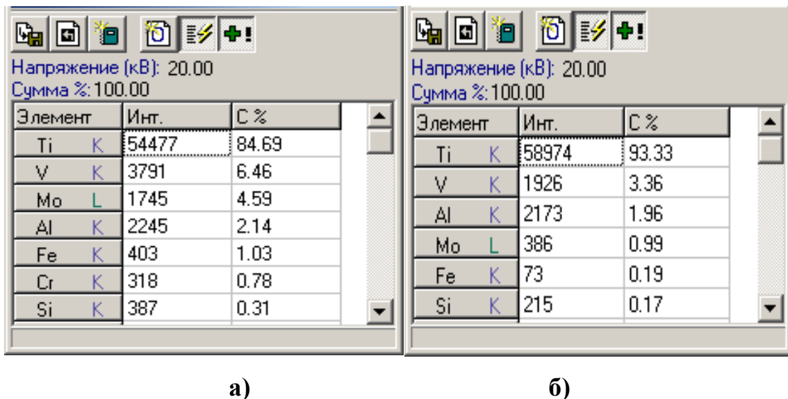
Рис. 1. Хімічний склад \alpha -фази (а) та \beta -фази (б) при гартуванні 850°C
