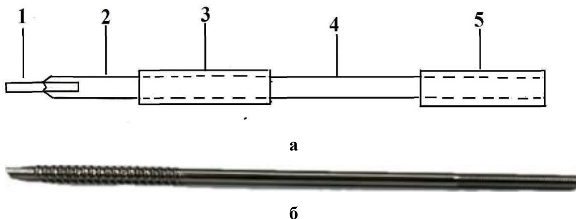
Рис. 1. Схематичне зображення стрижня для компресійного остеосинтеза переломів тіла ключиці (а) : 1- отвір для направляючої спиці, 2- свердло, 3- направляюча різьба, 4- тіло, 5- різьба для компресійної гайки; (б): натуральне зображення стрижня.
