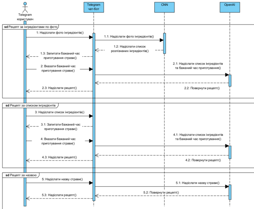
Рис. 2 Діаграма послідовності
