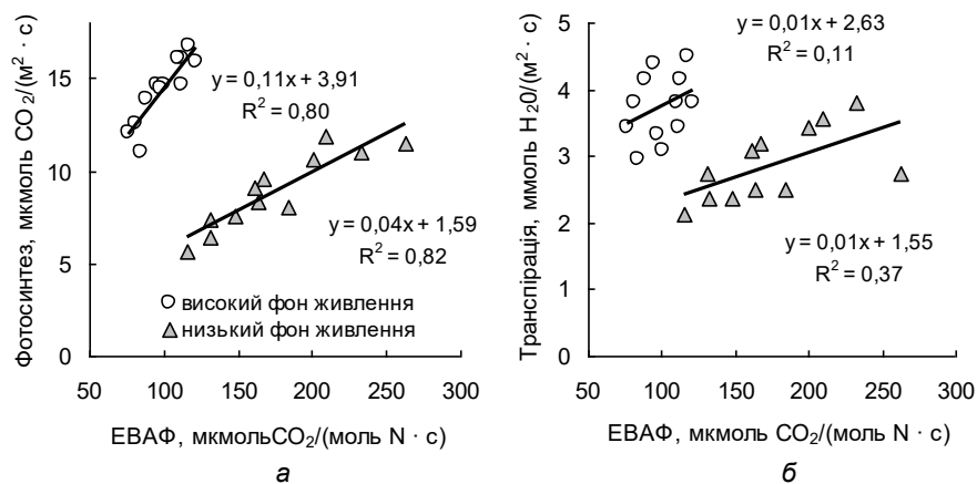
Рис. 1. Зв'язок між ефективністю використання азоту (ЕВАФ) та інтенсивністю фотосинтезу (а) і транспірації (б) листків пшениці різних сортів і умов мінерального живлення
