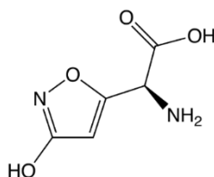
Рис. 12. Іботенова кислота
