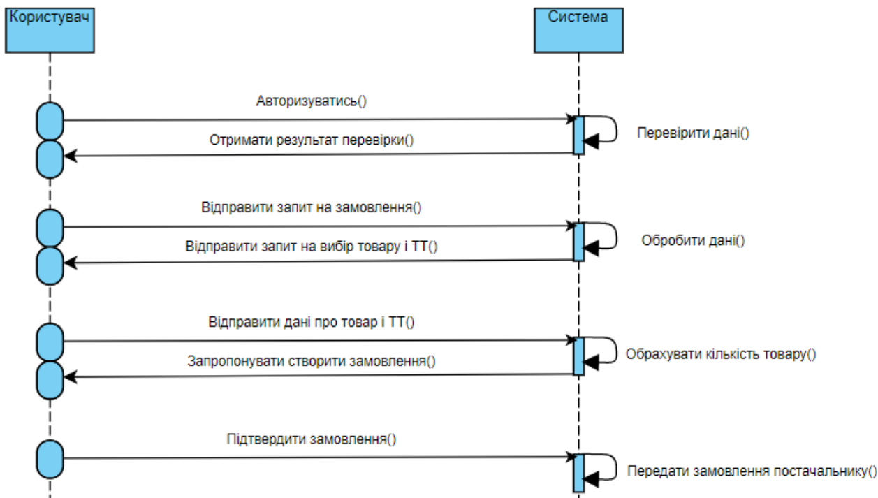
Рис. 1. Діаграма послідовності
