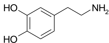
Рис. 4. Допамін
