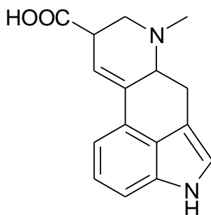
Рис. 7. Лізергінова кислота
