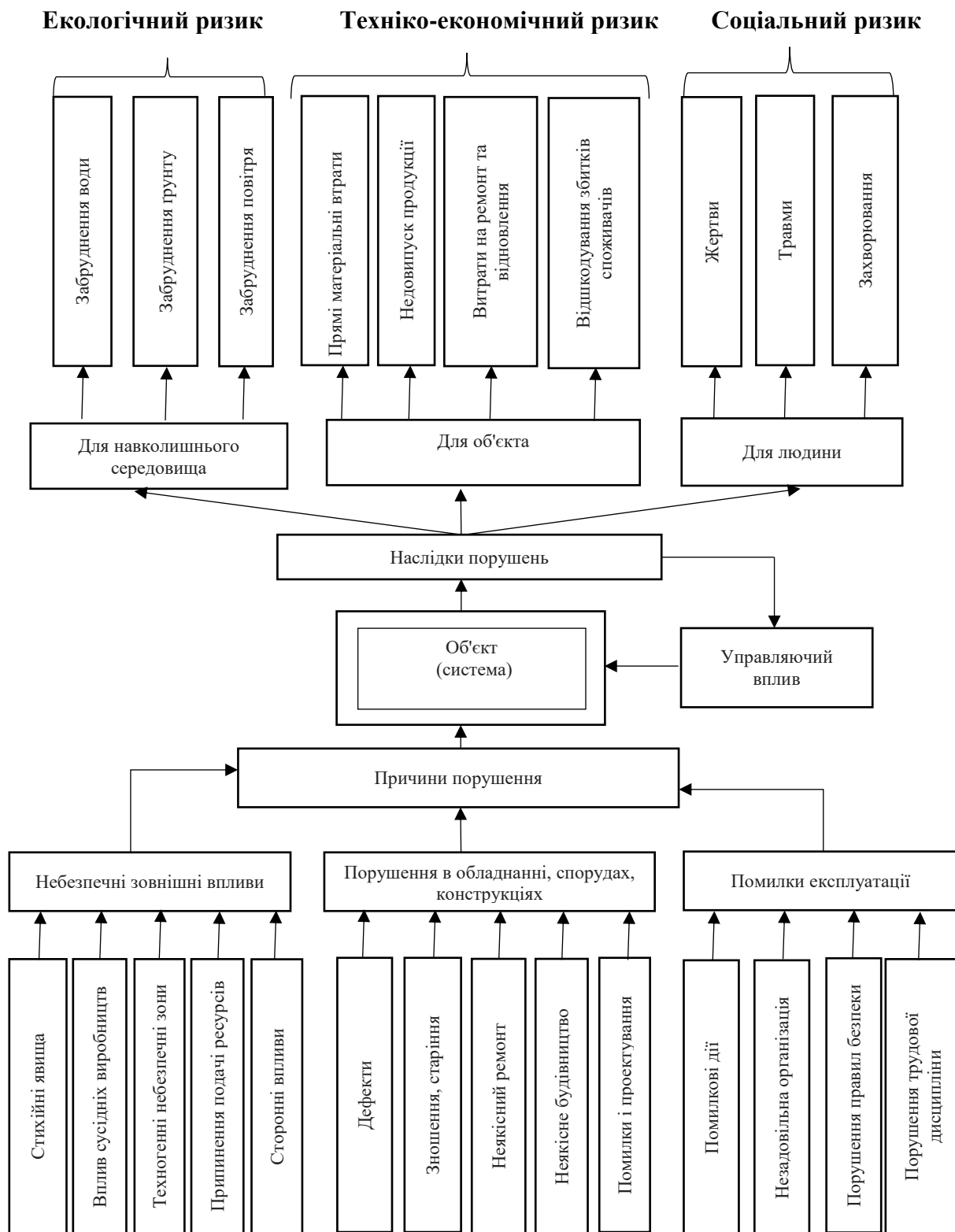
Рис. Функціональна модель промислової безпеки об'єктів електроенергетики при технологічних порушеннях
