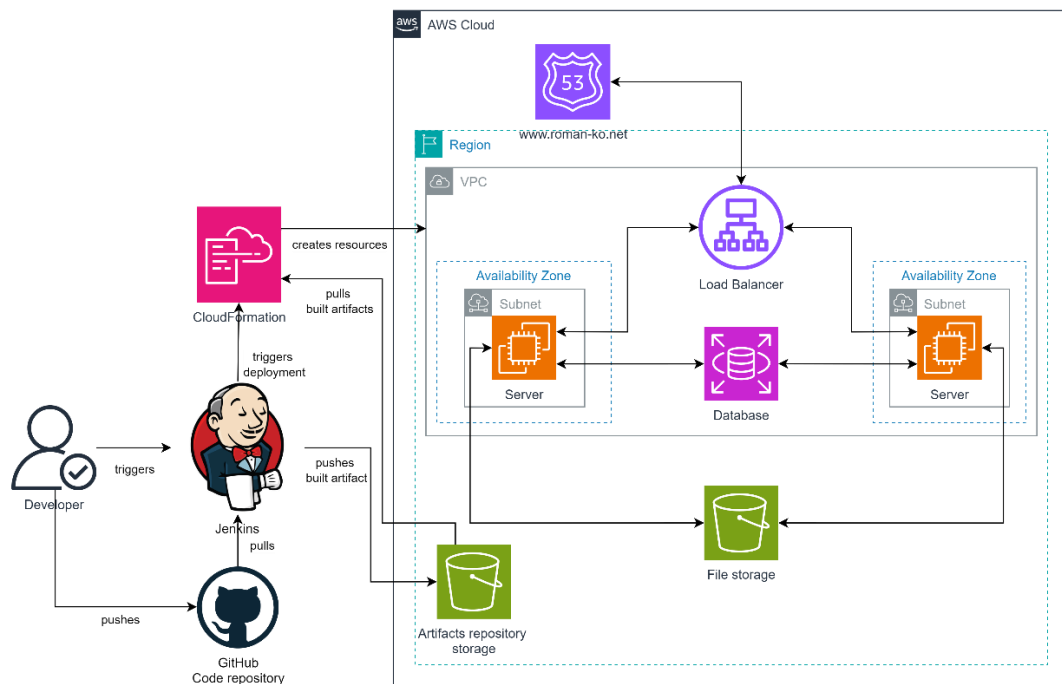
Рис. 2. Модель CI/CD процесів автоматизованої системи моніторингу стану дерев
