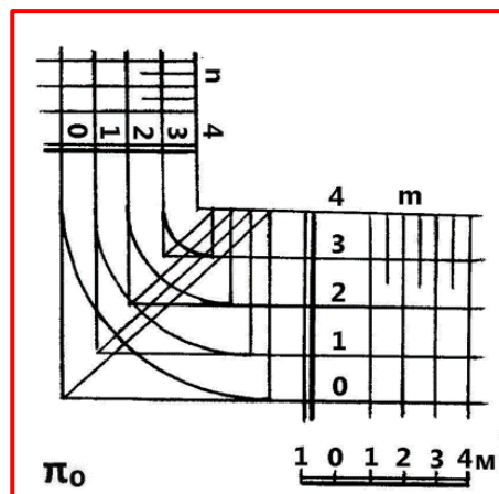
Рис. 2. Спряження укосів при їх різних ухилах поверхнею еліптичного конуса
