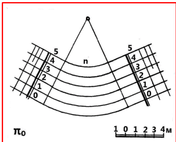
Рис. 1. Спряження укосів за їх однаковими ухилами поверхнею конуса обертання
