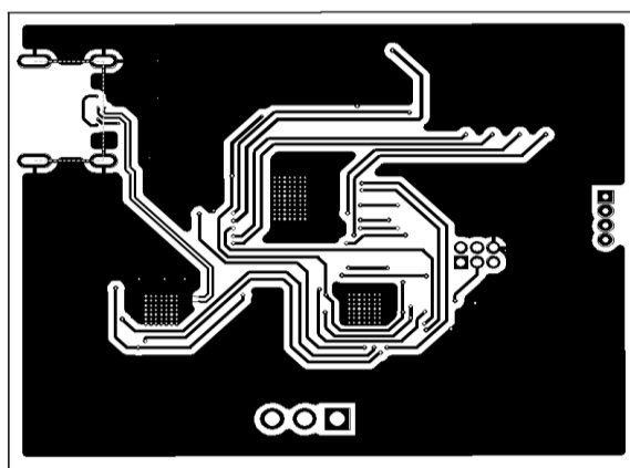
Рис. 1. Нижній шар друкованої плати
