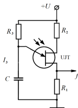
Рис. 3. Схема фотодатчика на одному ОПТ
