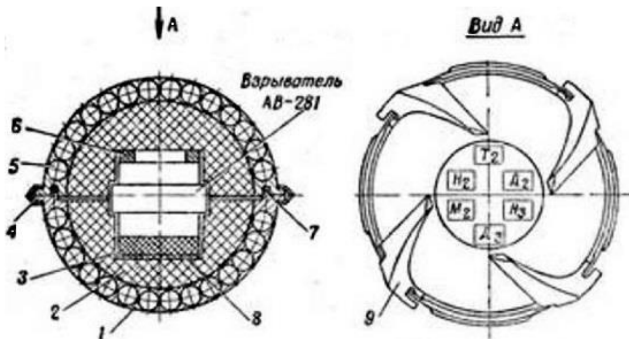
Рис. 2. Схематичне зображення кулькової осколкової авіабомби «ШОАБ-0,5»: 1. Полусфера; 2. Бойовий заряд (вибухова суміш ТГ-30/70); 3. Детонаторна шашка; 4. З'єднувальне кільце; 5. Стальна кулька; 6. Повстяна прокладка; 7. Гумове кільце; 8. Сукняна прокладка; 9 Приплив.
