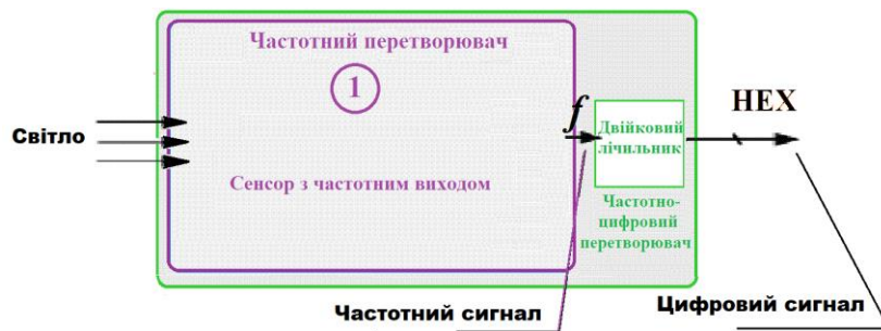
Рис. 2. Цифровий датчик з частотним чутливим елементом, вихідним параметром якого є частота f
