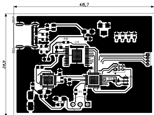
Рис. 2. Верхній шар друкованої плати
