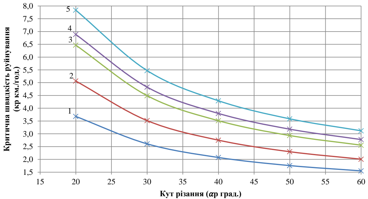
Рис. 2 Залежність критичної швидкості різання від кута різання ножа 1 – твердий супісок; 2 – напівтвердий суглинок; 3 – тугопластична глина; 4 – твердий суглинок; 5 – напівтверда глина.
