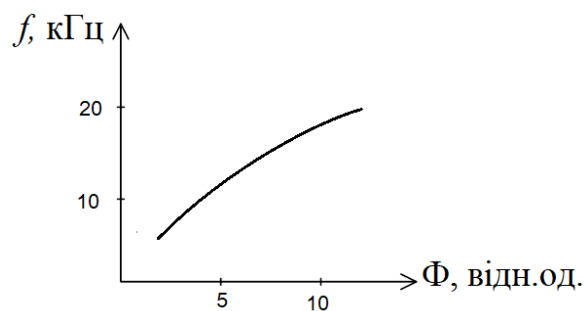
Рис. 4. Вихідна характеристика фотодатчика на одному ОПТ
