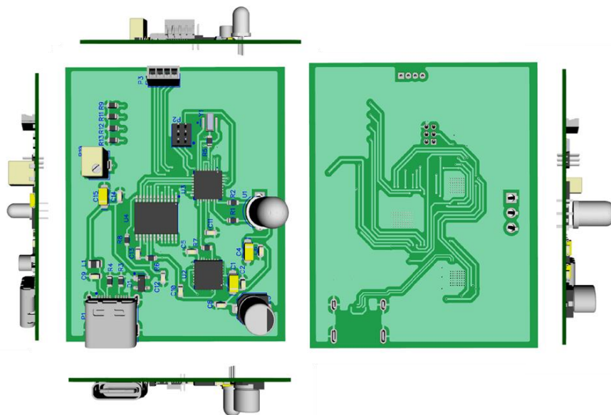
Рис. 3. 3D модель плати контролера двигуна
