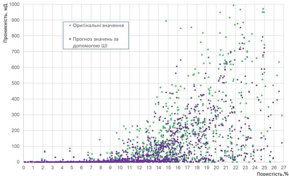
Рис. 2. Зіставлення значень абсолютної проникності та коефіцієнта пористості та значень абсолютної проникності та пористості, згенеровані за допомогою ШІ на основі геофізичних досліджень
