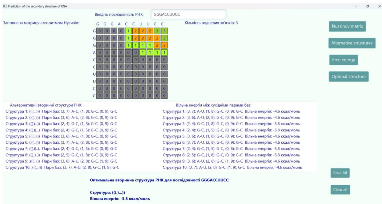
Рис. 4. Кінцевий результат з визначеною оптимальною вторинною структурою
