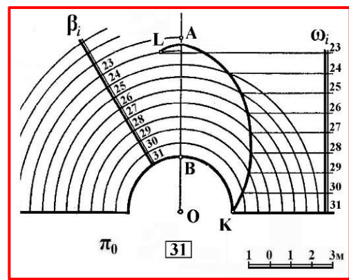
Рис. 6. Перетин укосів \gamma і \beta , коли ухил укосу \nu менший за ухил укосу \beta
