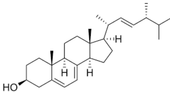
Рис. 5. Ергостерол
