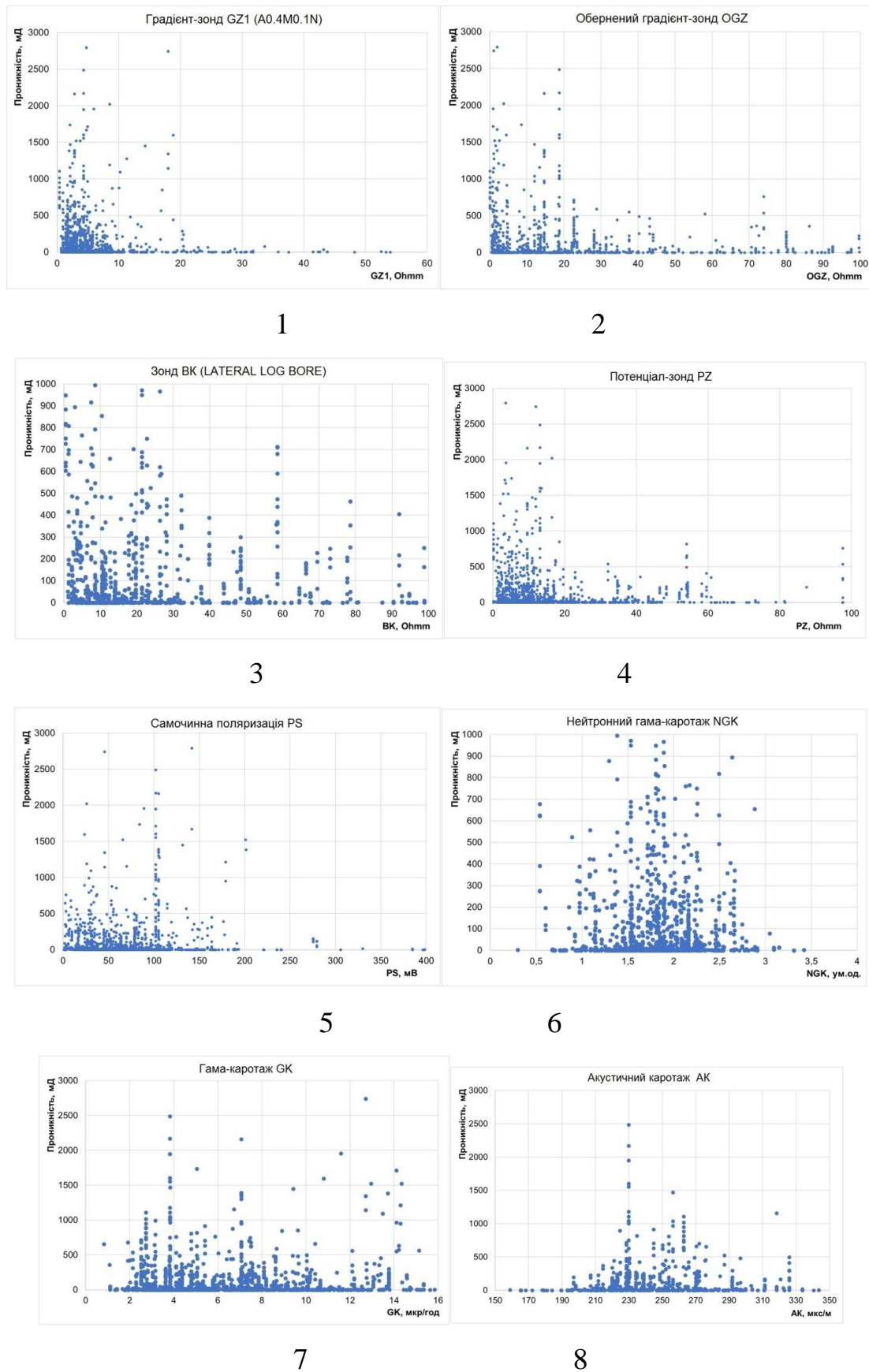
Рис. 1. Зіставлення значень абсолютної проникності та даних геофізичних методів (1-4 – покази електричних зондів, 5 – самочинна поляризація, 6 – нейтронний гама-каротаж, 7 – гама-каротаж, 8 – акустичний каротаж)
