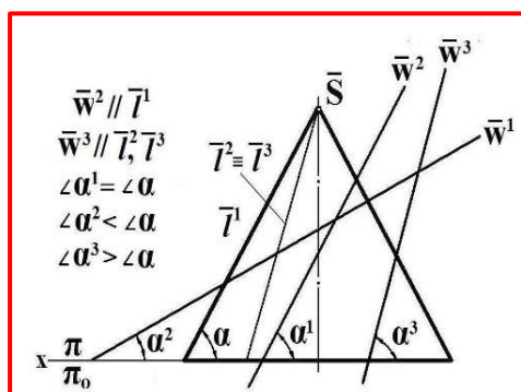
Рис. 3. Перетин поверхні конуса січними площинами w^1, w^2, w^3
