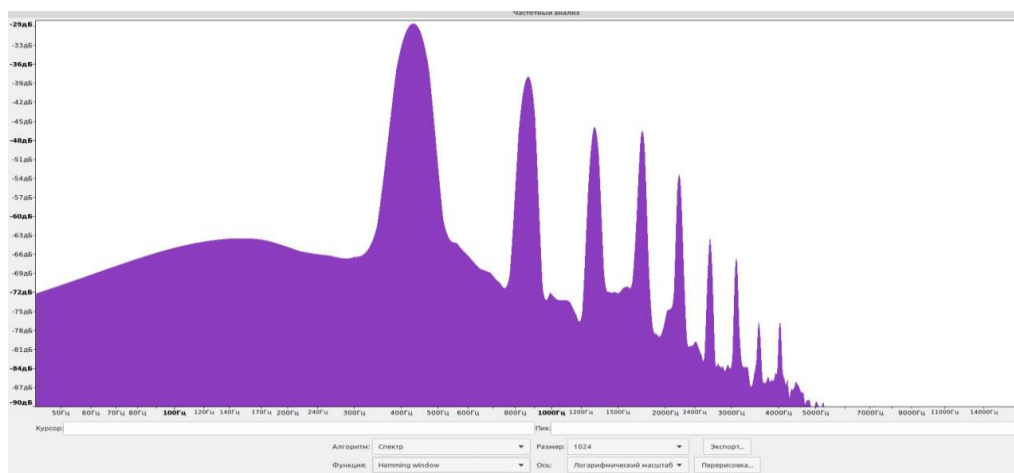
Мал. 2. Приклад спектра простої ноти, що виконується на гітарі.
