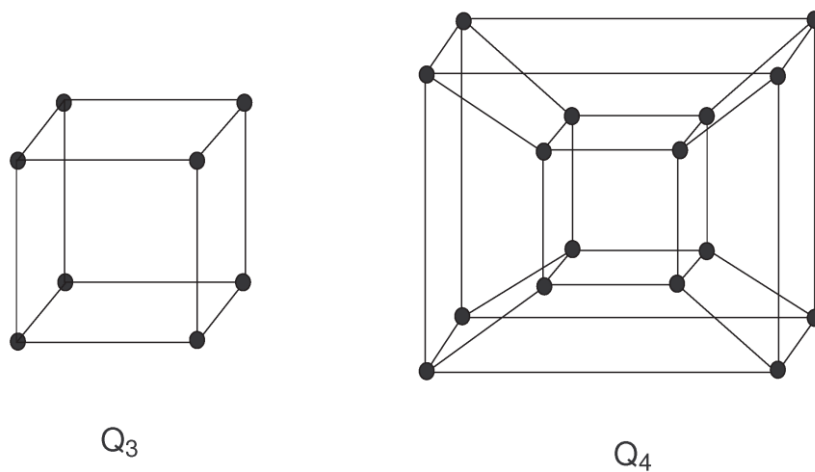
Рис. 1. Графи гіперкуба Q_3 та Q_4
