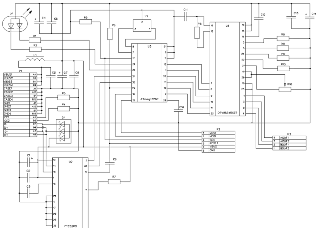
Схема 1. Схема електрична принципова драйвера двигуна
