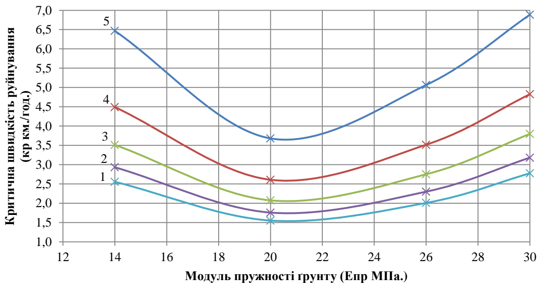
Рис. 3 Залежність критичної швидкості різання від модуля пружності ґрунту при різних кутах різання 1 – α р =60°; 2 – α р =50°; 3 – α р =40°; 4 – α р =30°; 5 – α р =20°;
