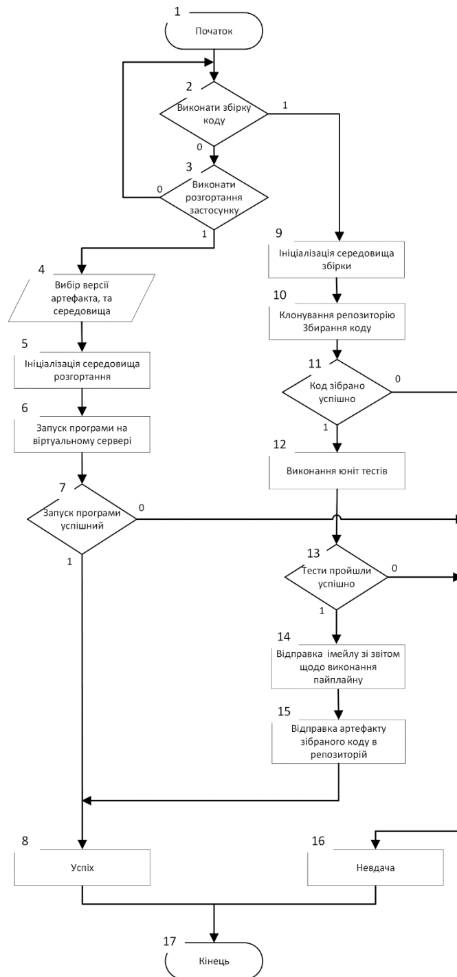
Рис. 1. Алгоритм роботи CI/CD системи моніторингу стану дерев
