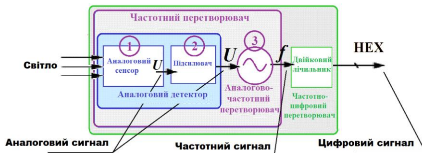
Рис. 1. Цифровий світловий датчик з аналоговим чутливим елементом, в якому вхідним параметром є напруга U
