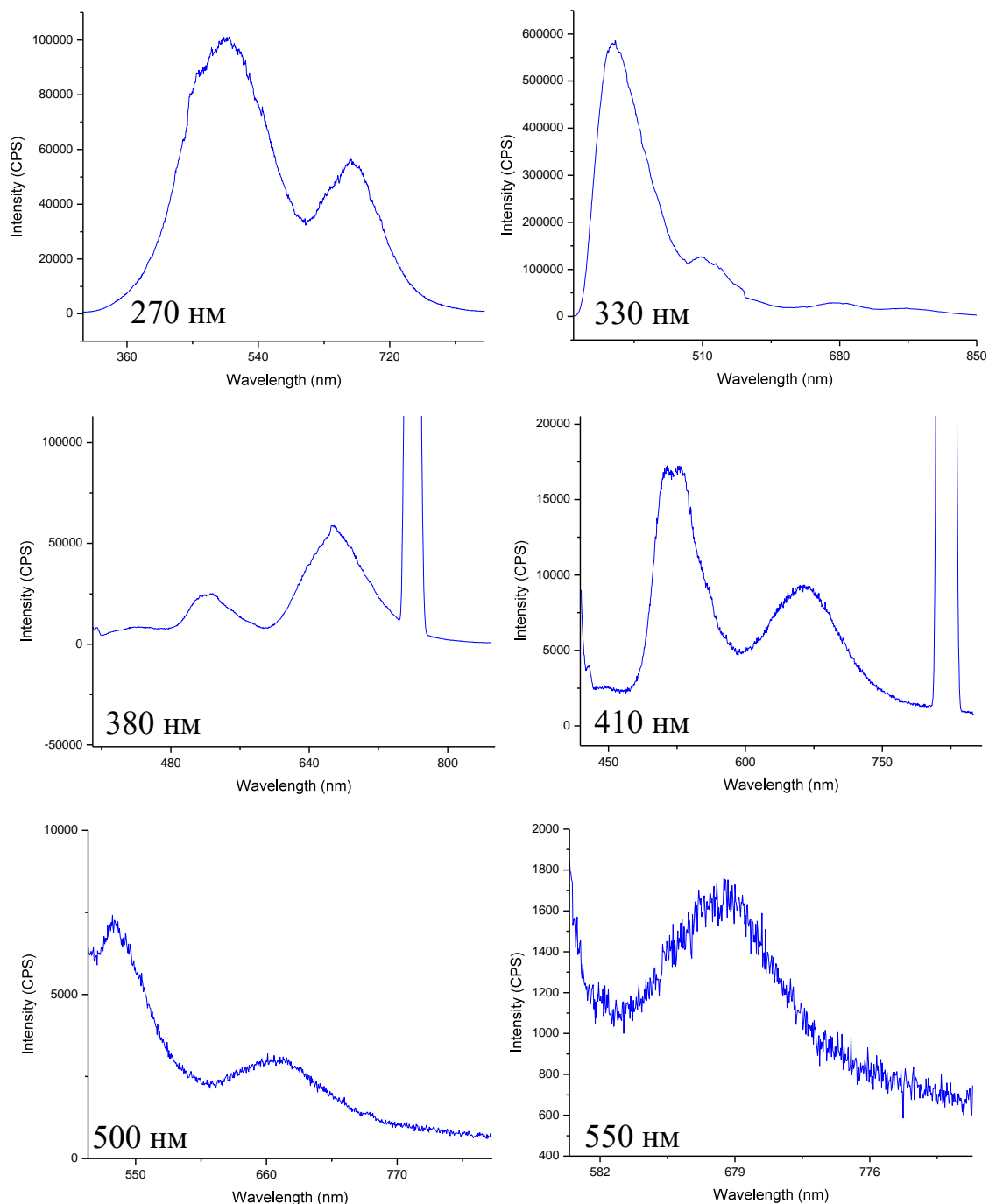
Рис. 4. Спектри люмінесценції шару напильня в наносекундному розряді з мідними електродами в повітрі атмосферного тиску при збудженні різними довжинами хвиль випромінювання.
