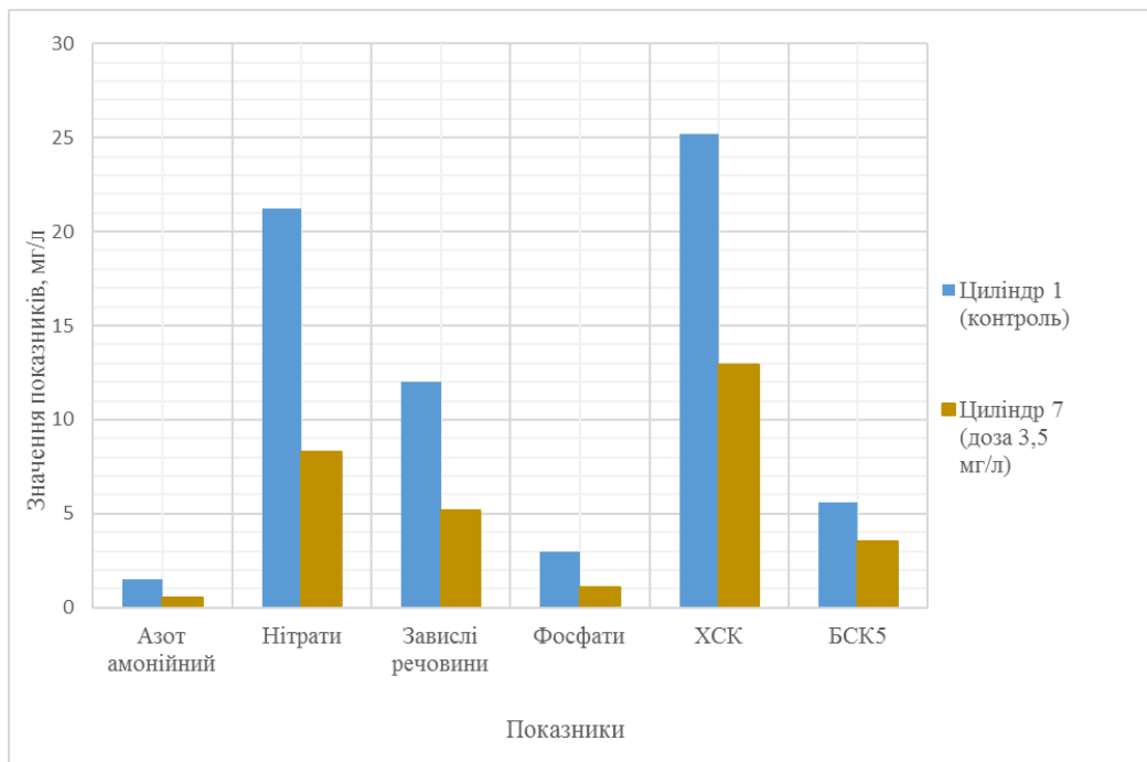
Рис. 1. Діаграма показників хімічних аналізів вод контрольної проби та за обробки озонно-кисневою сумішшю з дозою озону 3,5 мг/дм 3
