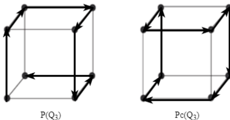
Рис. 2. Гамільтоновий шлях P(Q_3) та гамільтоновий цикл Pc(Q_3)
