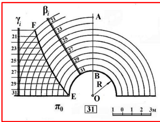
Рис. 5. Перетин укосів \gamma і \beta , що мають однакові ухили
