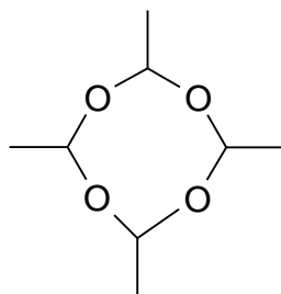
Рис. 7. Метальдегід
