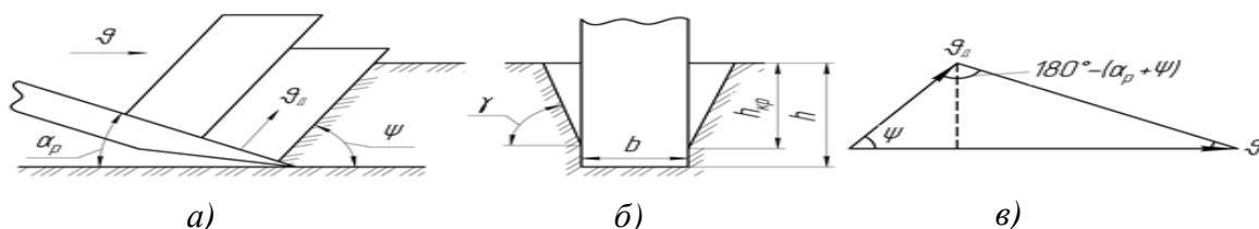
Рис. 1 Схема утворення елементної стружки в процесі різання ґрунту елементарним ножем: а) – у профільній площині; б) – у фронтальній площині; в – план швидкостей
