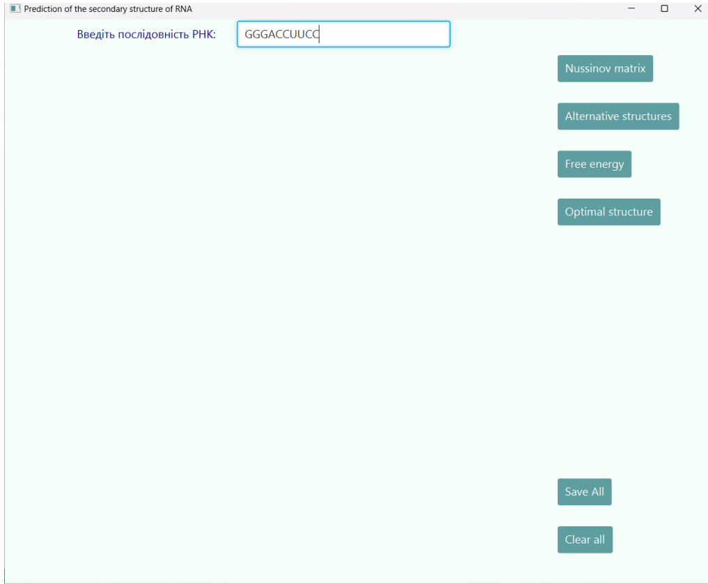
Рис. 1. Введення користувачем послідовності РНК
