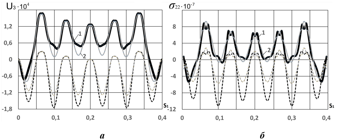
Рисунок 2. Максимальні величини прогинів і напружень в серединних поверхнях несучих шарів при жорсткому затисненні торців структури:
