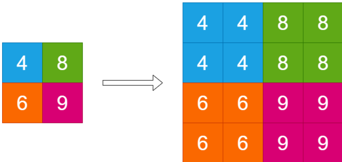
Рис. 1 – Інтерполяція методом найближчого сусіда
