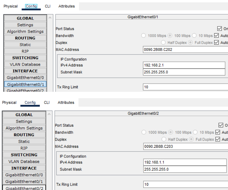
Рисунок 3 – Мережні налаштування ISP
