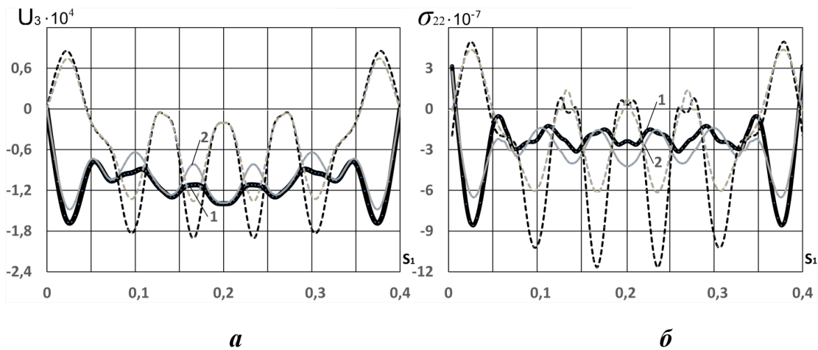
Рисунок 3. Максимальні величини прогинів і напружень в серединних поверхнях несучих шарів при шарнірному затисненні торців структури:
