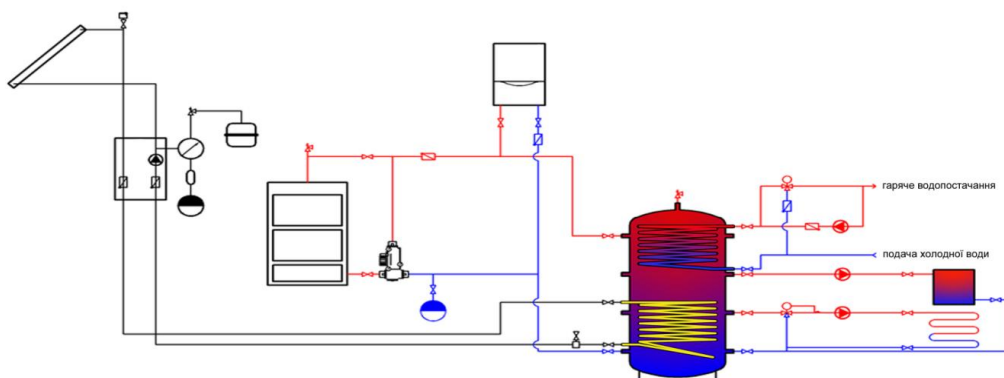
Рис. 1. Схема зберігання теплової енергії у водяних баках.
