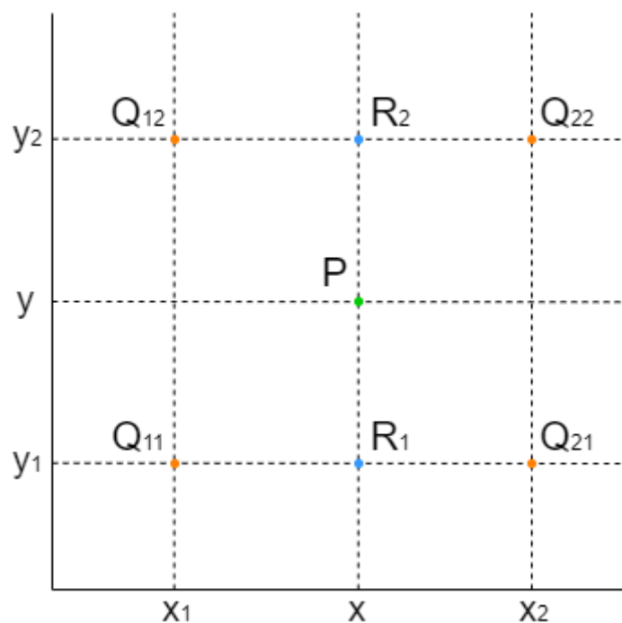
Рис. 2 – Приклад білінійної інтерполяції
