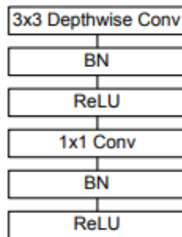
Рисунок 1. Базовий блок моделі MobileNet
