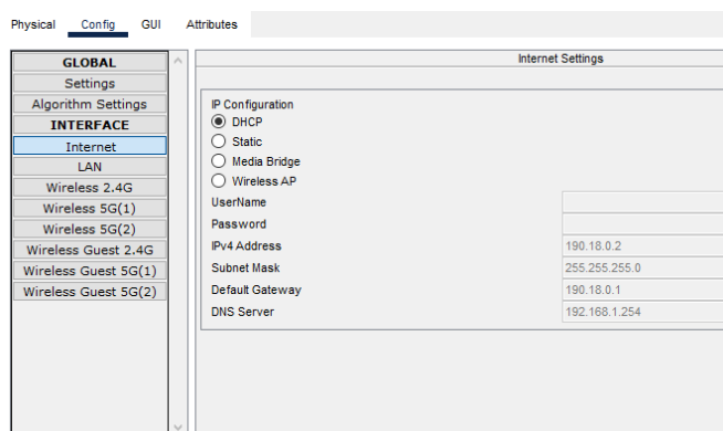
Рисунок 2 – Вікно налаштувань інтерфейсу Internet на маршрутизаторі
