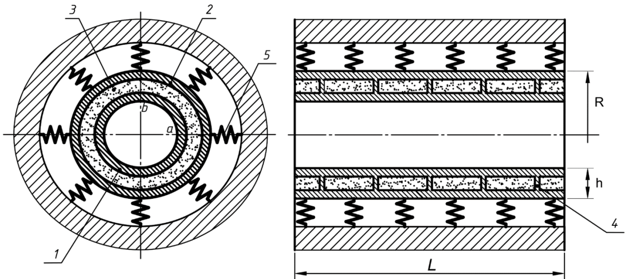
Рисунок 1. Конструкція тришарової циліндричної оболонки кругового та еліптичного перерізу з полімерним заповнювачем армованим ребрами: 1 - внутрішній шар; 2 – зовнішній шар; 3 - полімерний заповнювач (t); 4 - армуючі ребра (j); 5 – пружне середовище Вінклера
