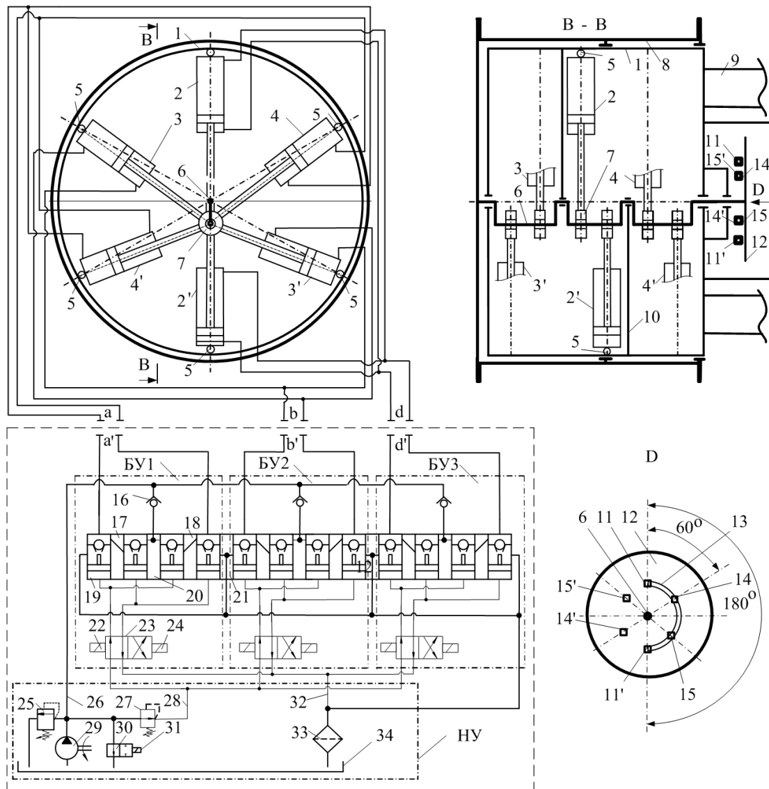
Рис. 4. Структурна схема мотора на базі силових циліндрів і клапанно-золотникової гідроапаратури для управління ними
