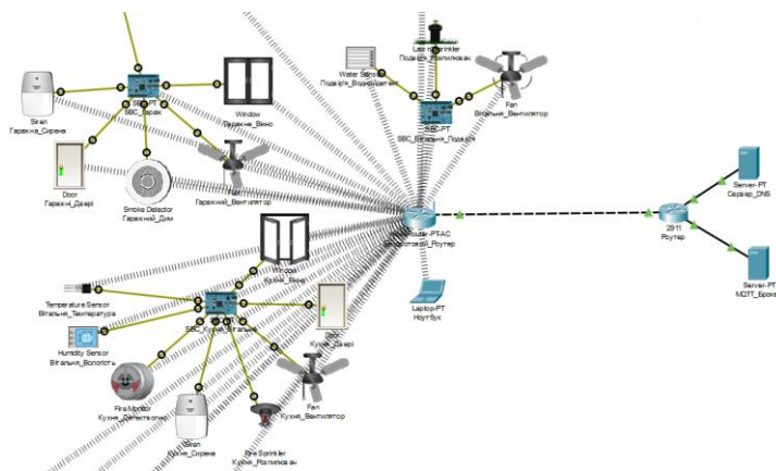
Рисунок 1 – Структура системи «розумного будинку»
