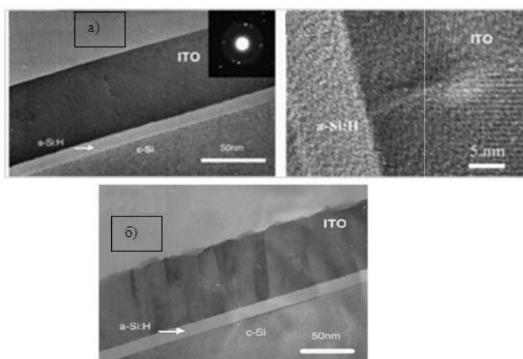
Рис. 3. Изображения, полученные методом просвечивающей электронной микроскопии пленок ITO (а - на стекле) и ITO (б - на подложки кремния)
