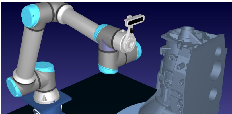
Рис. 1 Модель робота UR-10e з камерою машинного зору для контролю якості нанесення покриттів
