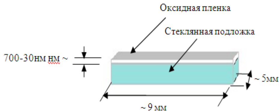
Рис. 5. Схема и характерные размеры образца
