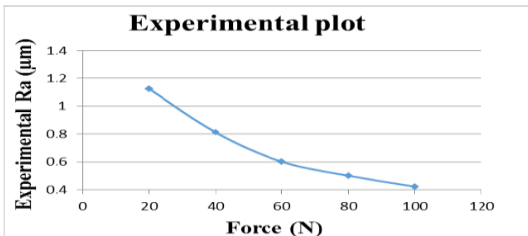
Рис. 2 – Графік шорсткості поверхні відповідно до тиску, прикладеного на розкочувальний ролик
