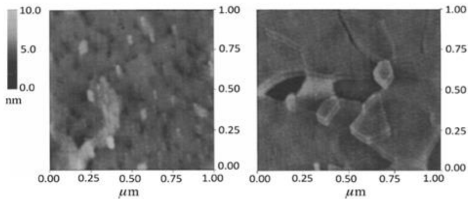
Рисунок. 4 Изображения пленок ИТО, осажденных при комнатной температуре на стеклянной подложке полученные методом атомной силовой микроскопии
