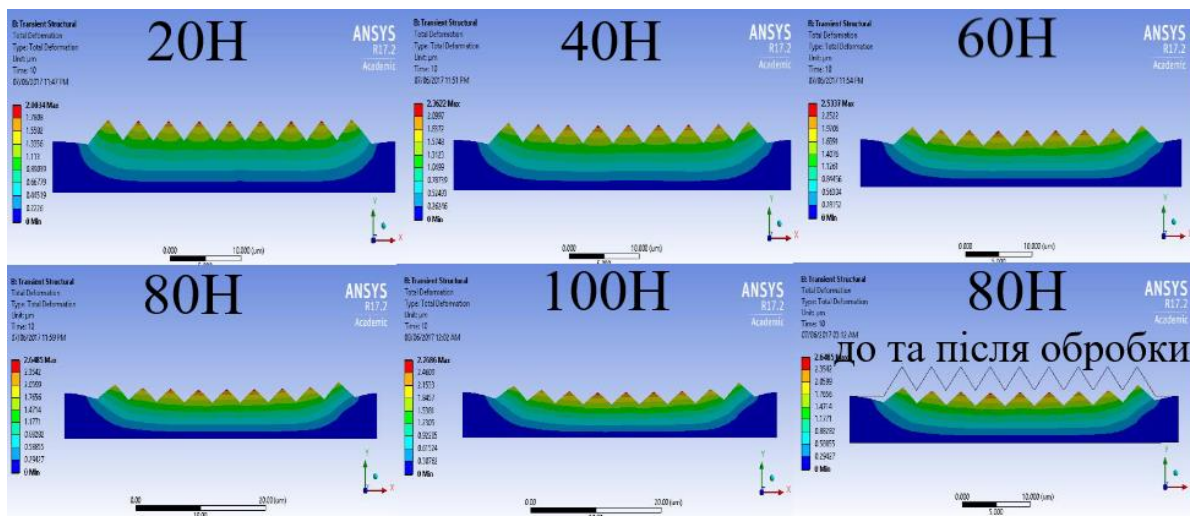
Рис. 1 – Показник шорсткості поверхні відповідно до тиску, прикладеного на розкочувальний ролик
