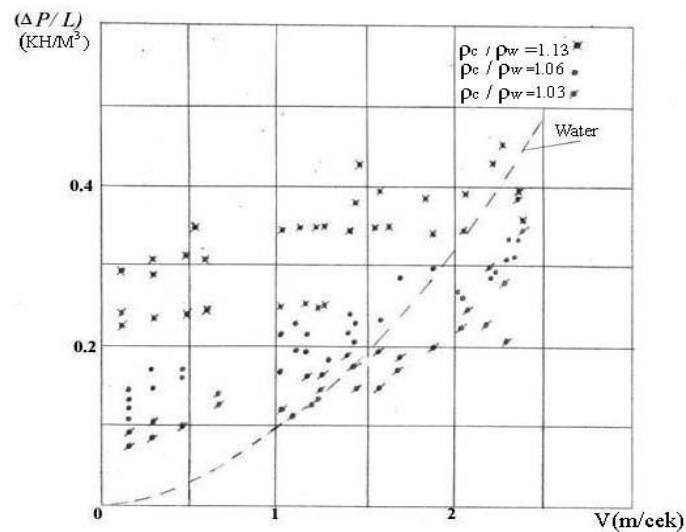
Рис. 1а. Залежність гідравлічних опорів капсульного потоку від V для першої серії дослідів [3].
