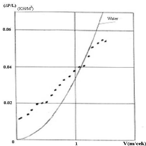
Рис. 1б. Залежність гідравлічних опорів капсульного потоку від V для другої серії дослідів [3].
