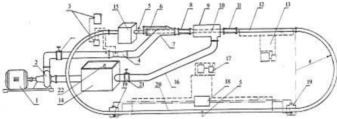
Рис. 2. Схема лабораторної кільцевої ежекторної установки D = 58 \text{ мм}
