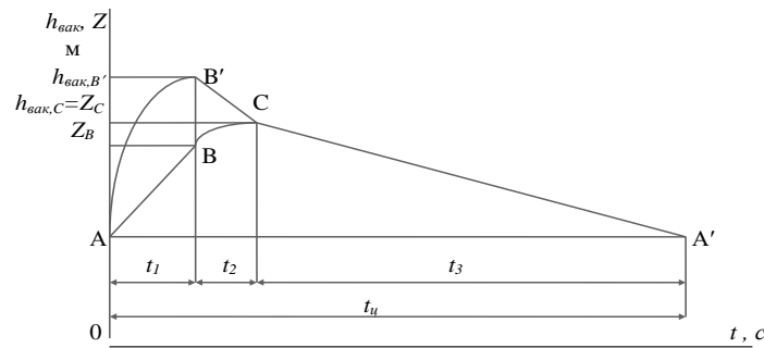
Рис. 2. Графік робочого циклу вакуумної установки
