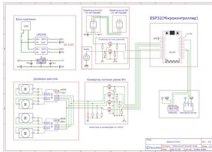
Рис. 1. Електрична схема
