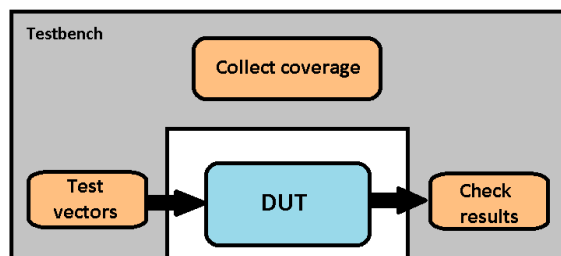
Рис. 1. Блок-схема тестового стенду для функціональної симуляції
