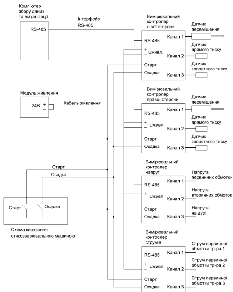
Рис. 1. Функціональна схема спеціалізованої комп'ютерної система контролю параметрів стикового зварювання
