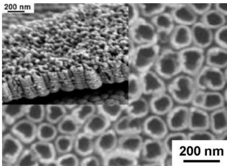
Рисунок. 1. Зображення нанотрубок \text{TiO}_2 .
