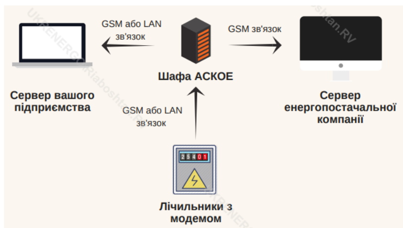
Рисунок 2. Структурна схема АСКОЕ
