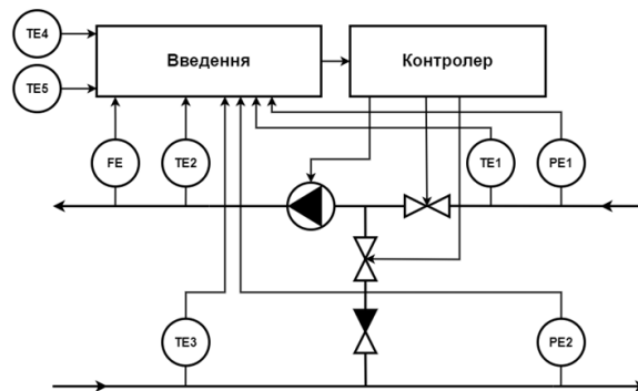
Рис. 1. Структурна схема ІТП
