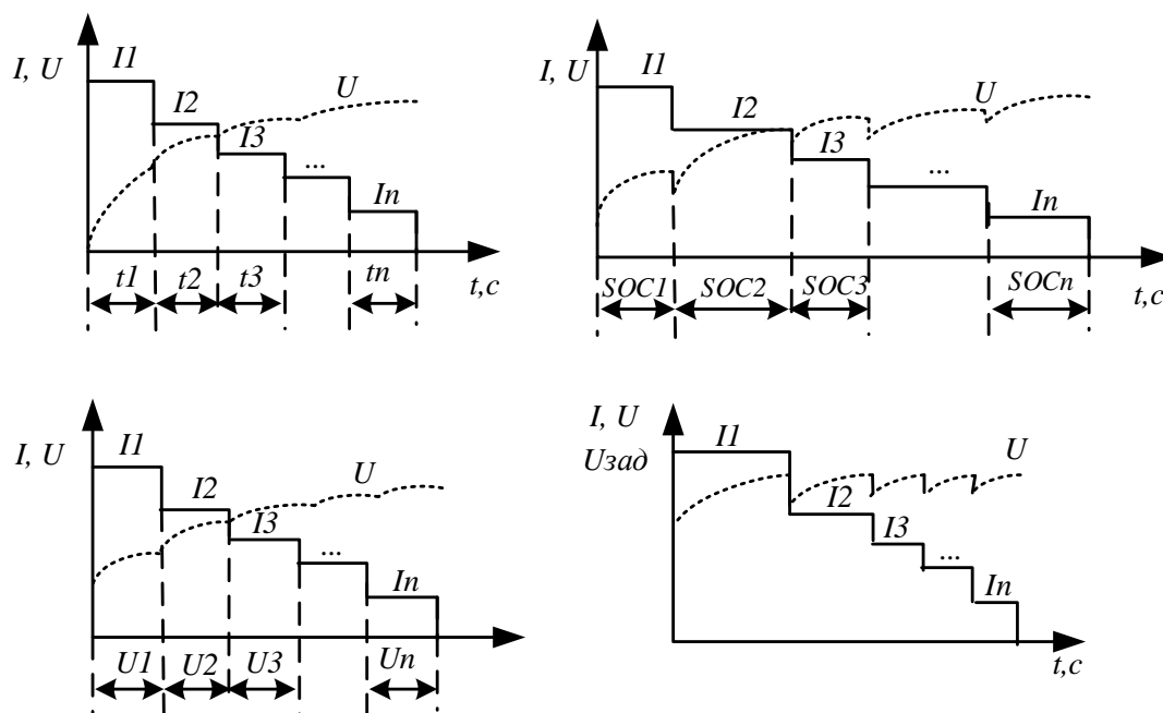
Рис. 1. Керування зарядом при переході з рівень на рівень на основі часу (а), SOC (б), порогової напруги (в), напруги відключення (г)
