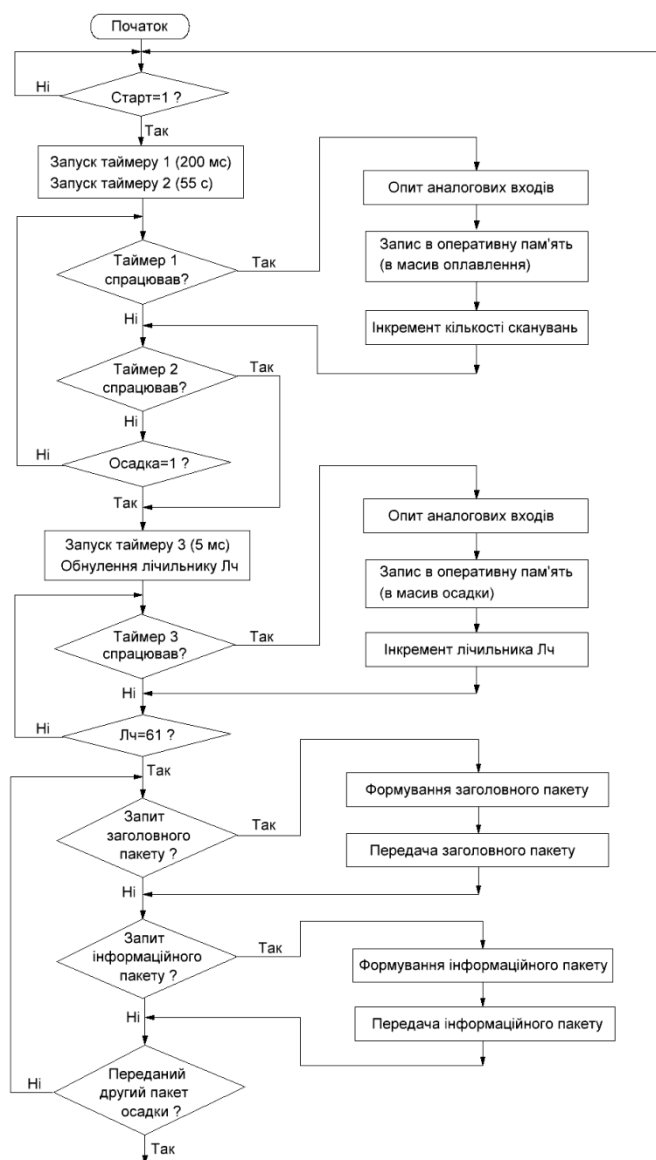
Рис. 2. Алгоритм програми вимірювального контролера
