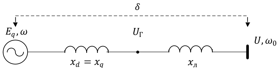
Рис. 1. Схема підключення ДРГ до шин енергосистеми
