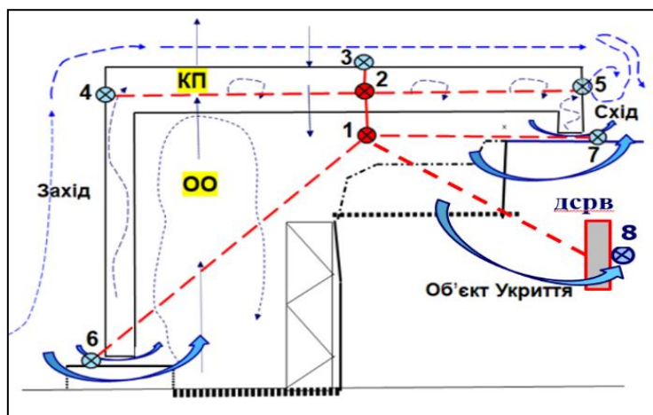
Рис. 1. Схема Нового Безпечного Конфайнменту та Об'єкту «Укриття» в поперечному перерізі. На рисунку: 1-8 вузли гідравлічної моделі НБК; 1 і 2—основний і кільцевий об'єми НБК; малі об'ємні стрілки - протікання повітря в місцях ущільнення мембран, великі – крізь будівельні конструкції під західною та східною стінами НБК
