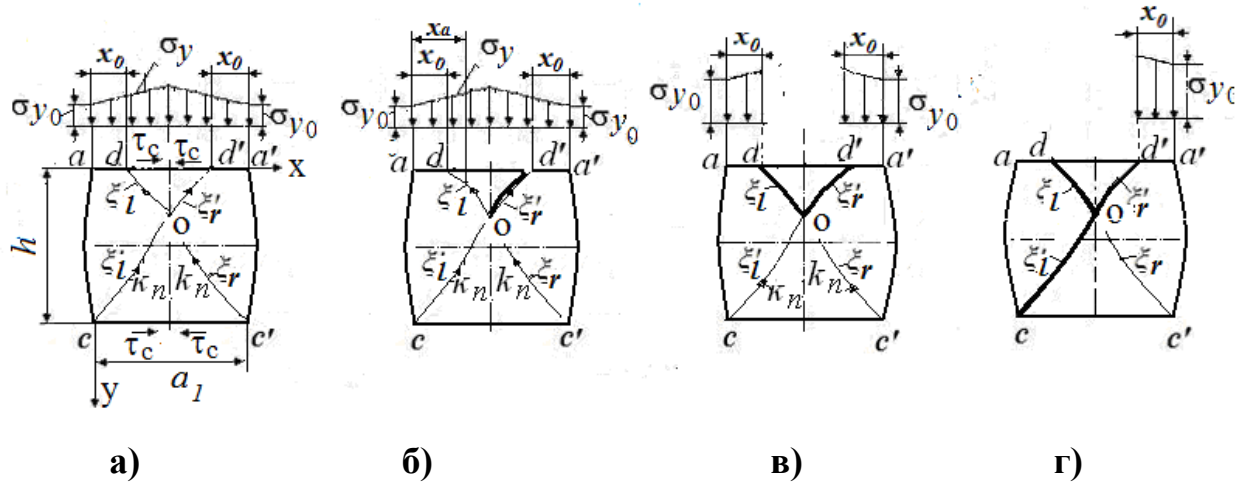
Рисунок 1 – Схема утворення клиновидної форми руйнування зразка гірських порід при його стисканні:
