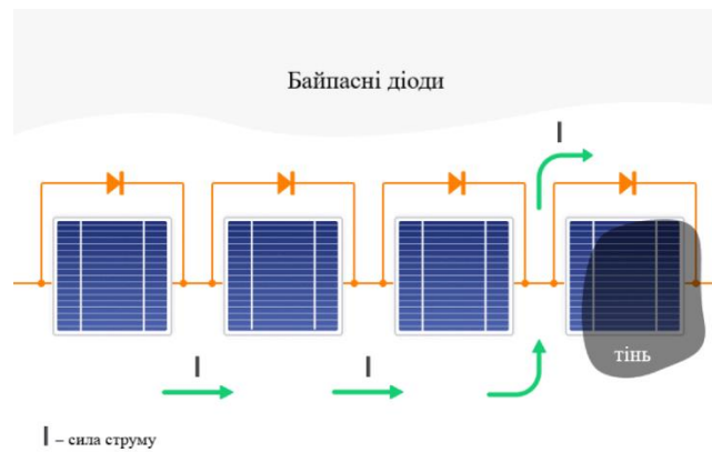
Рис. 1. Схема з байпасними діодами
