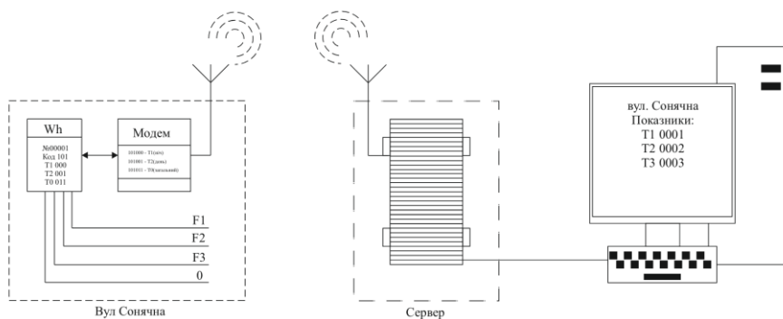
Рисунок 7. Принцип передачі даних методом індивідуального модему
