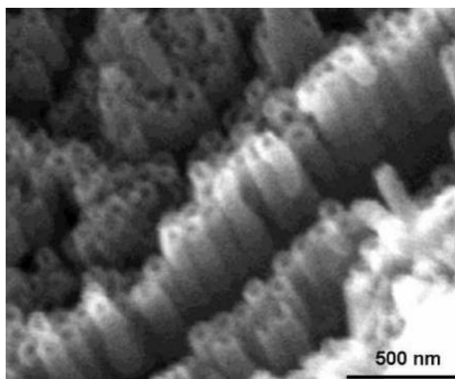
Рисунок. 2. Зображення наночастинок рутилу \text{TiO}_2 в форматі 3D: наностержні сферична частинка сформована з наностержнів рутилу.
