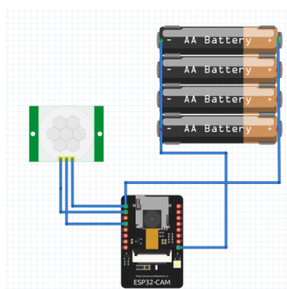
Рис. 1. Схема з'єднання спеціалізованої комп'ютерної система «розумного» домофону
