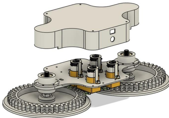
Рис. 2. Тривимірна модель збірки
