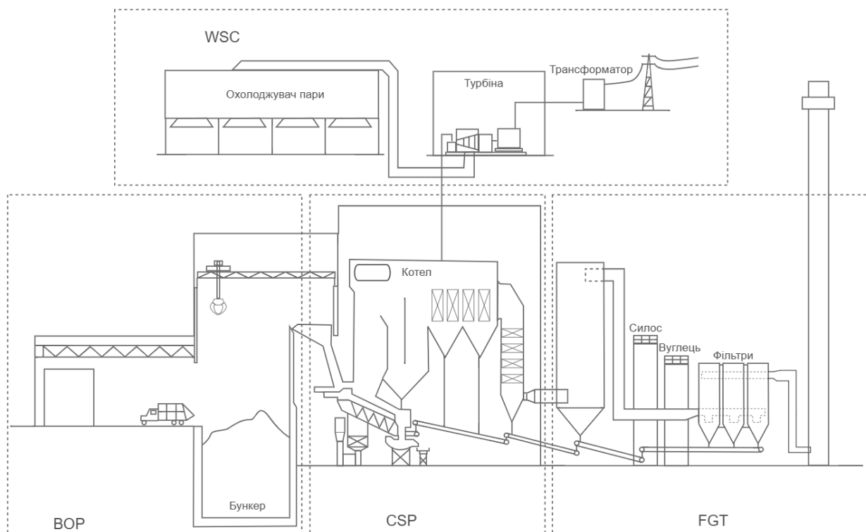
Рис. 1. Процес спалювання твердих побутових відходів
