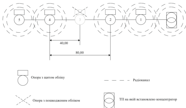
Рисунок 5. Аварійний режим роботи ZigBee системи
