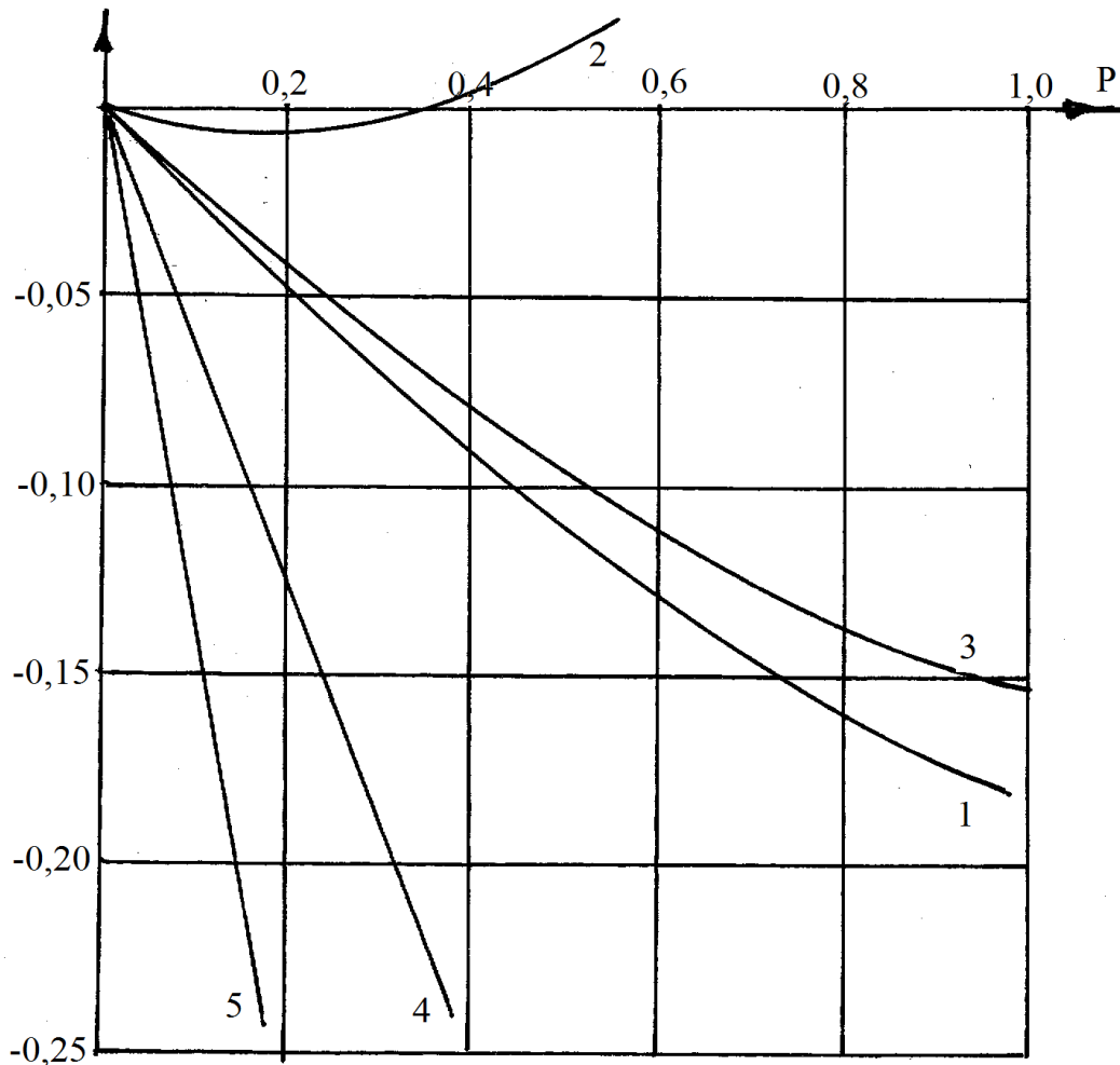
Рис. 2. Результати розрахунку коренів характеристичного рівняння
