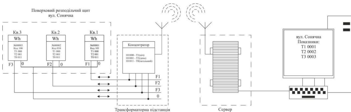
Рисунок 3. Принцип роботи PLC- системи
