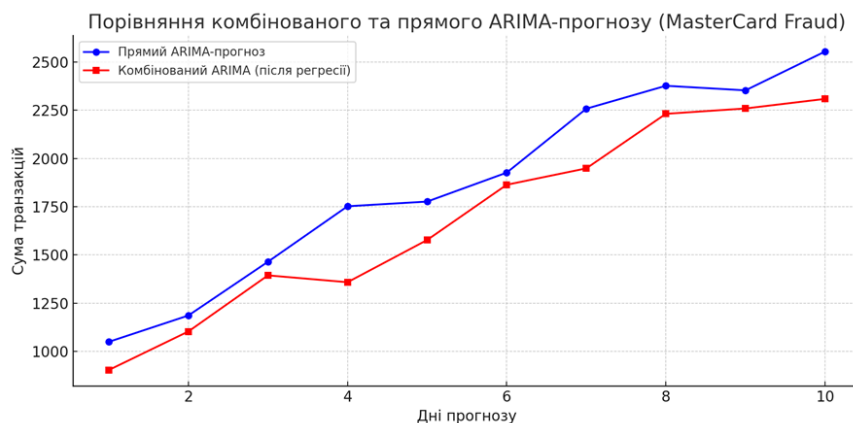
Рис. 2. Порівняння комбінованого та прямого ARIMA-прогнозу
