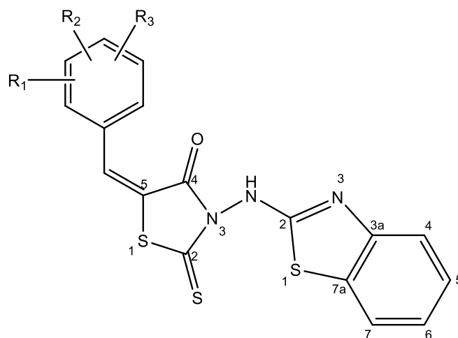
Рис. 1. Різноміснені 5-ариліденопохідні 3-(бензтіазол-2-іламіно)-2-тіоксо-4-тіазолідону
