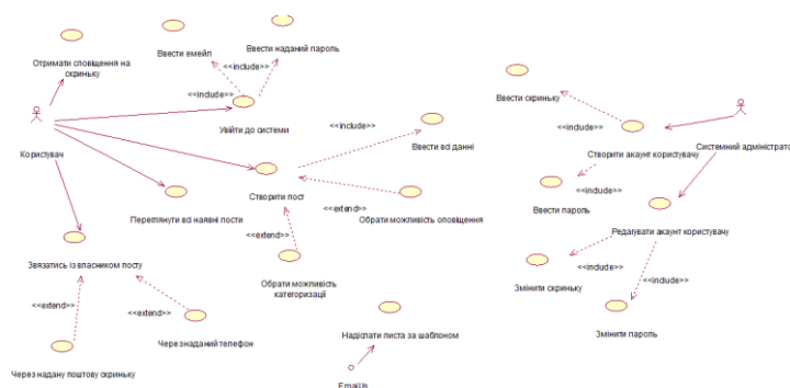
Рис. 1. Діаграма варіантів використання
