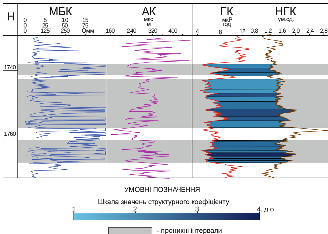
Рис. 1 – Прогнозна модель структурної неоднорідності геологічного розрізу інтервалу продуктивного горизонту P_3 нижньопермських відкладів Гнідинцівського НГКР, розкритого св. №173
