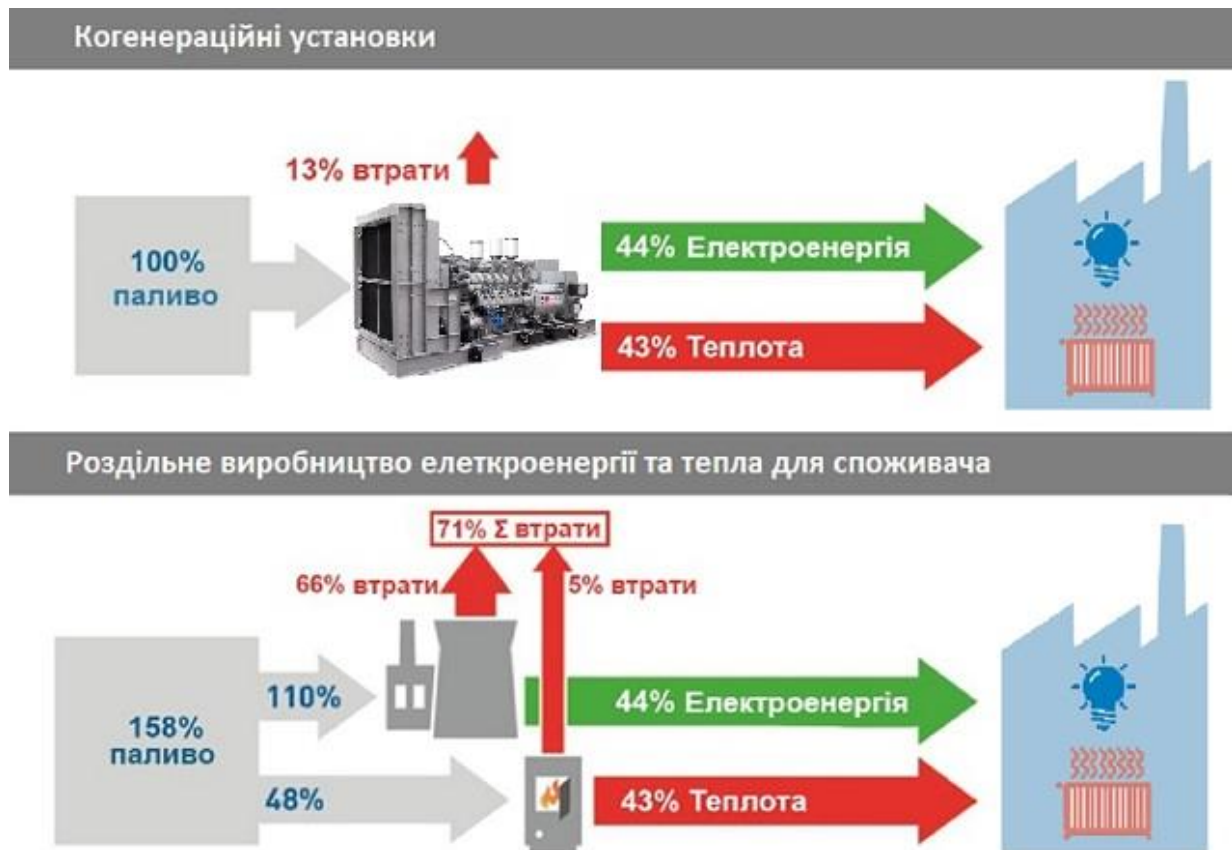
Рис. 1. Економічність використання когенераційною установки
