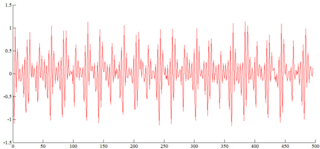
Рисунок 3. Часова реалізація змінної «u», отримана за допомогою комп'ютерної моделі аналогової схеми
