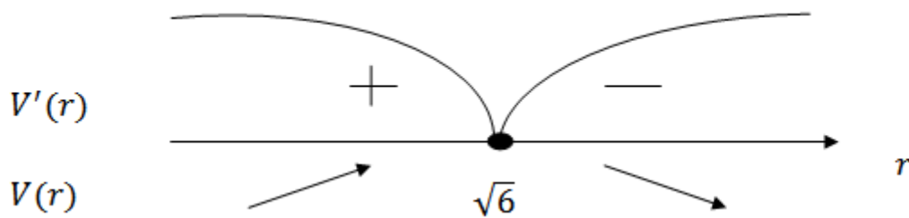
Рис. 2. Аналіз поведінки функції, похідної функції в критичній точці
