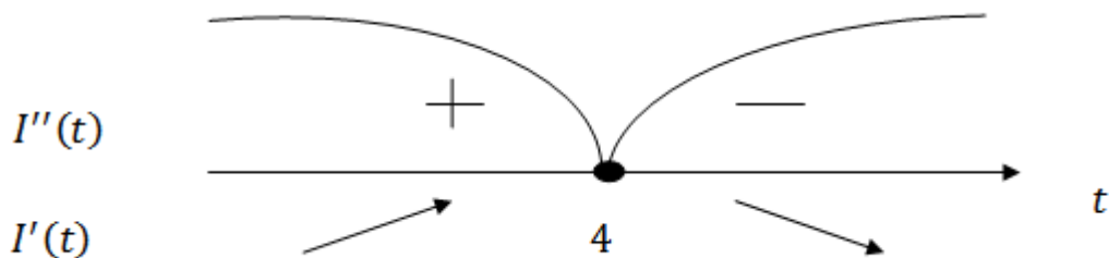
Рис. 3. Аналіз поведінки функції, похідної функції в критичній точці
