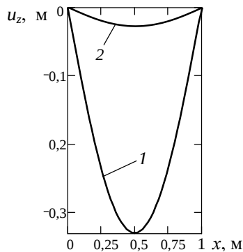
Рис. 2. Розподіл вздовж осі x переміщень u_z покриття
