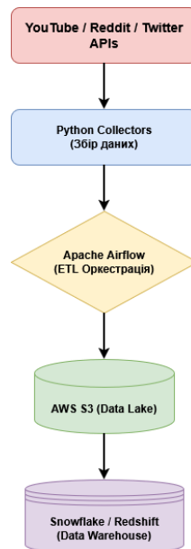
Рис. 1. Архітектура масштабованої системи збору великих даних
