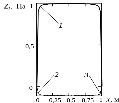
Рис. 1. Розподіл вздовж осі x нормальних напружень Z_z по поверхнях першого шару
